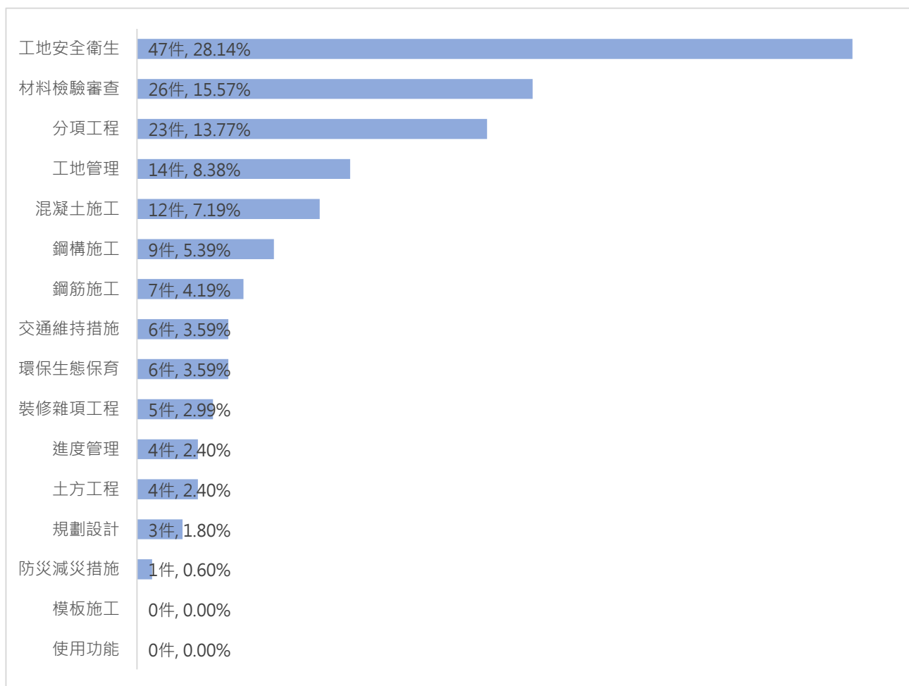
圖 3 110 年 1~2 月份施工查核「施工品質」缺失統計圖
