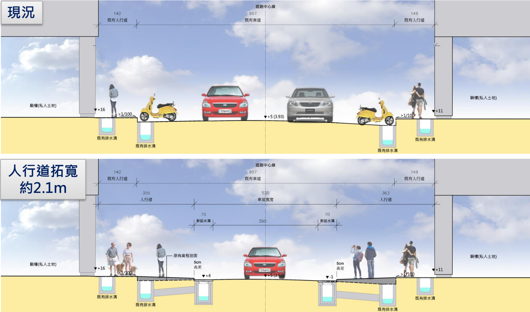
剖面示意圖
