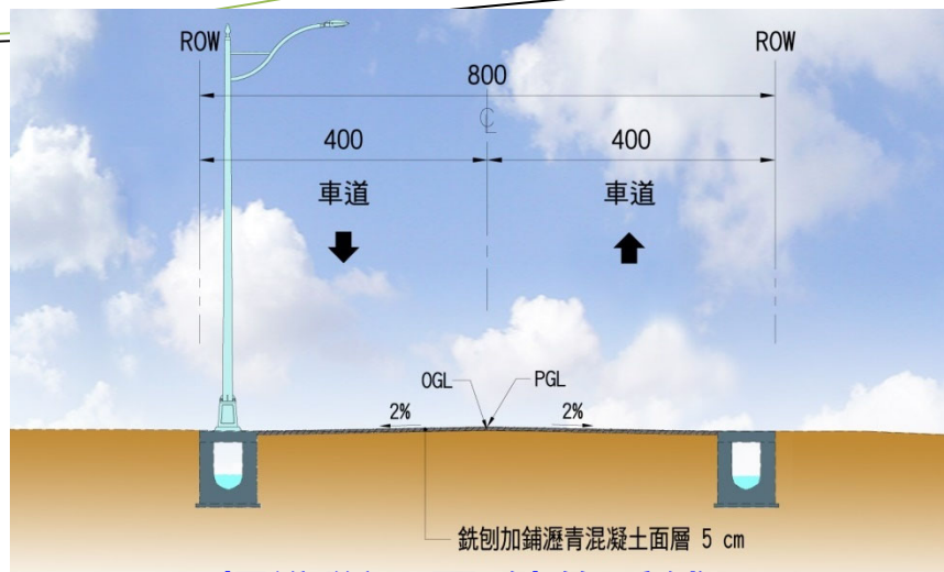
標準斷面圖(銑刨重鋪)
