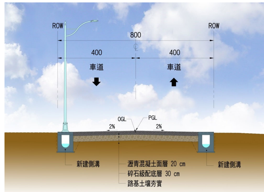
標準斷面圖(新築道路)
