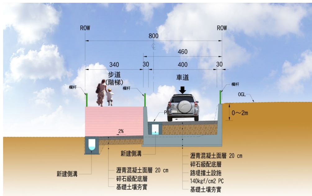
標準斷面圖(配合現況出入高程)
