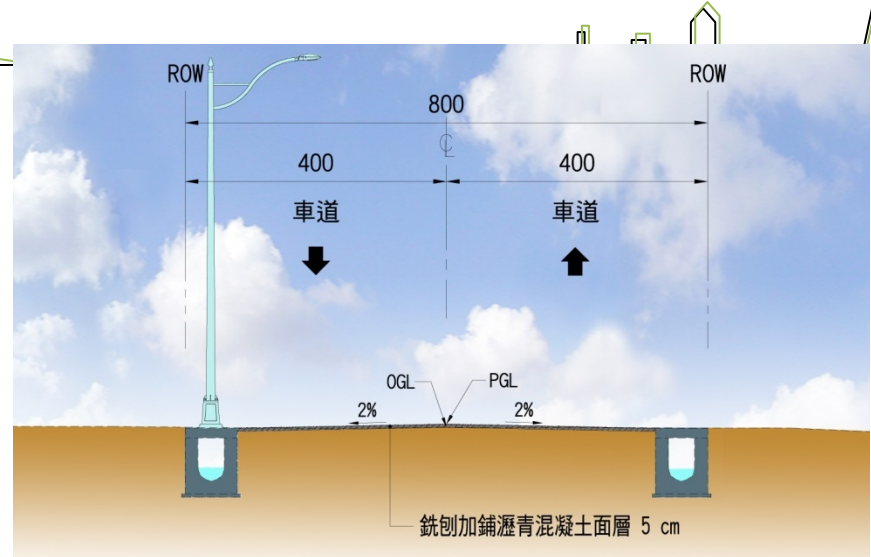
標準斷面圖(銑鉋重鋪)
