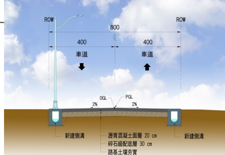
標準斷面圖(新築道路)
