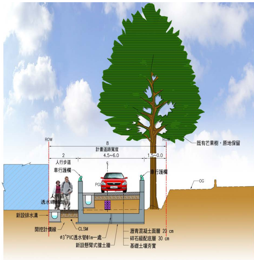
OK+044 ~ OK+065.6 方案一標準斷面圖(一般道路)
