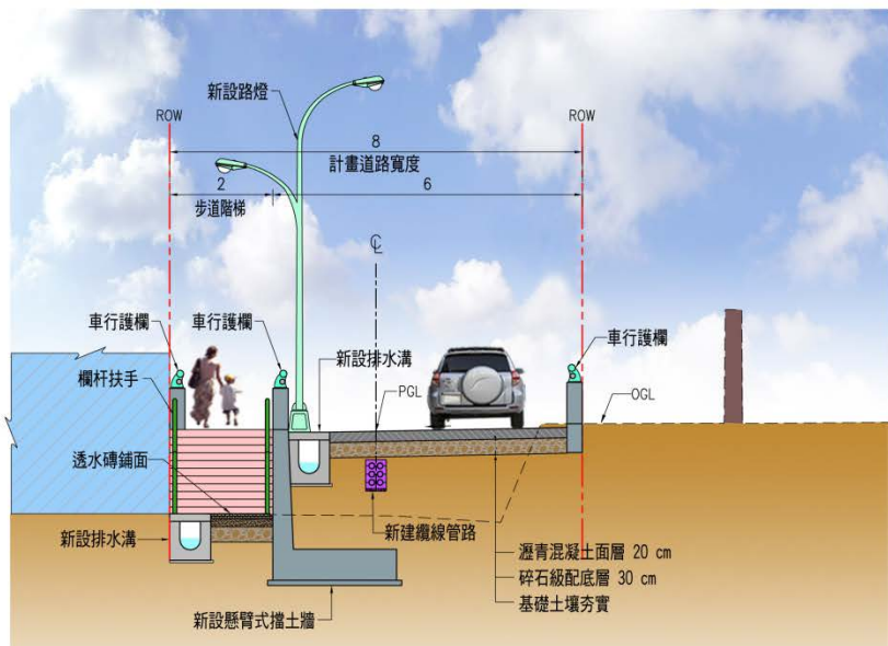
OK+044 ~ OK+065.6 方案一標準斷面圖(一般道路)
