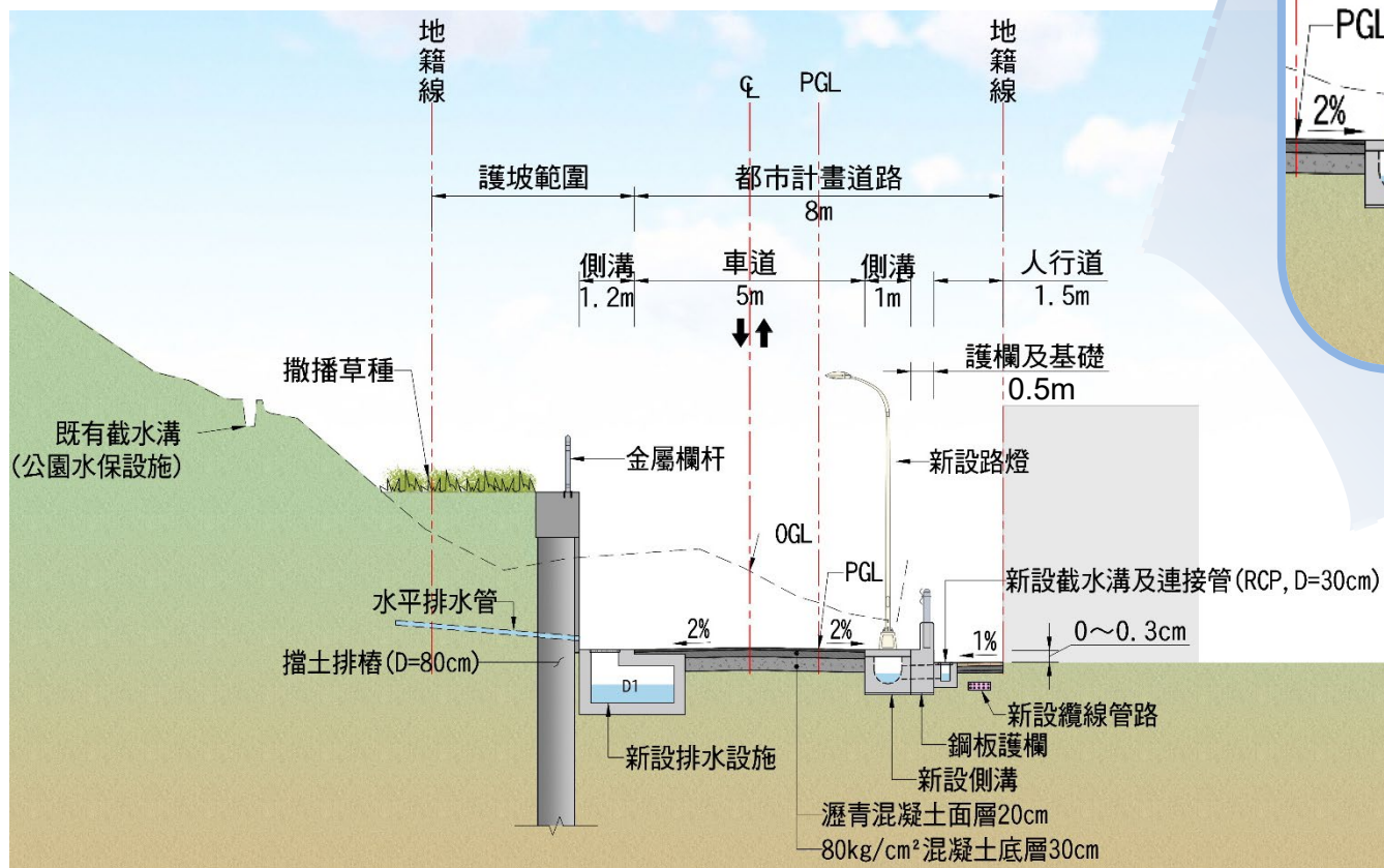
標準橫斷面圖(二)
