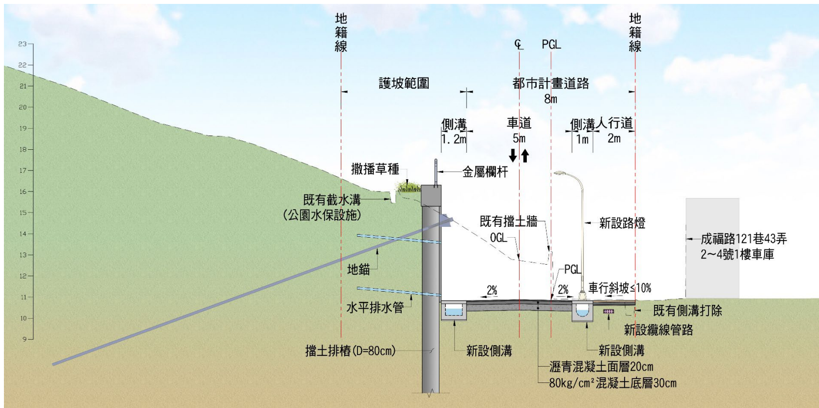
標準橫斷面圖 (一)
