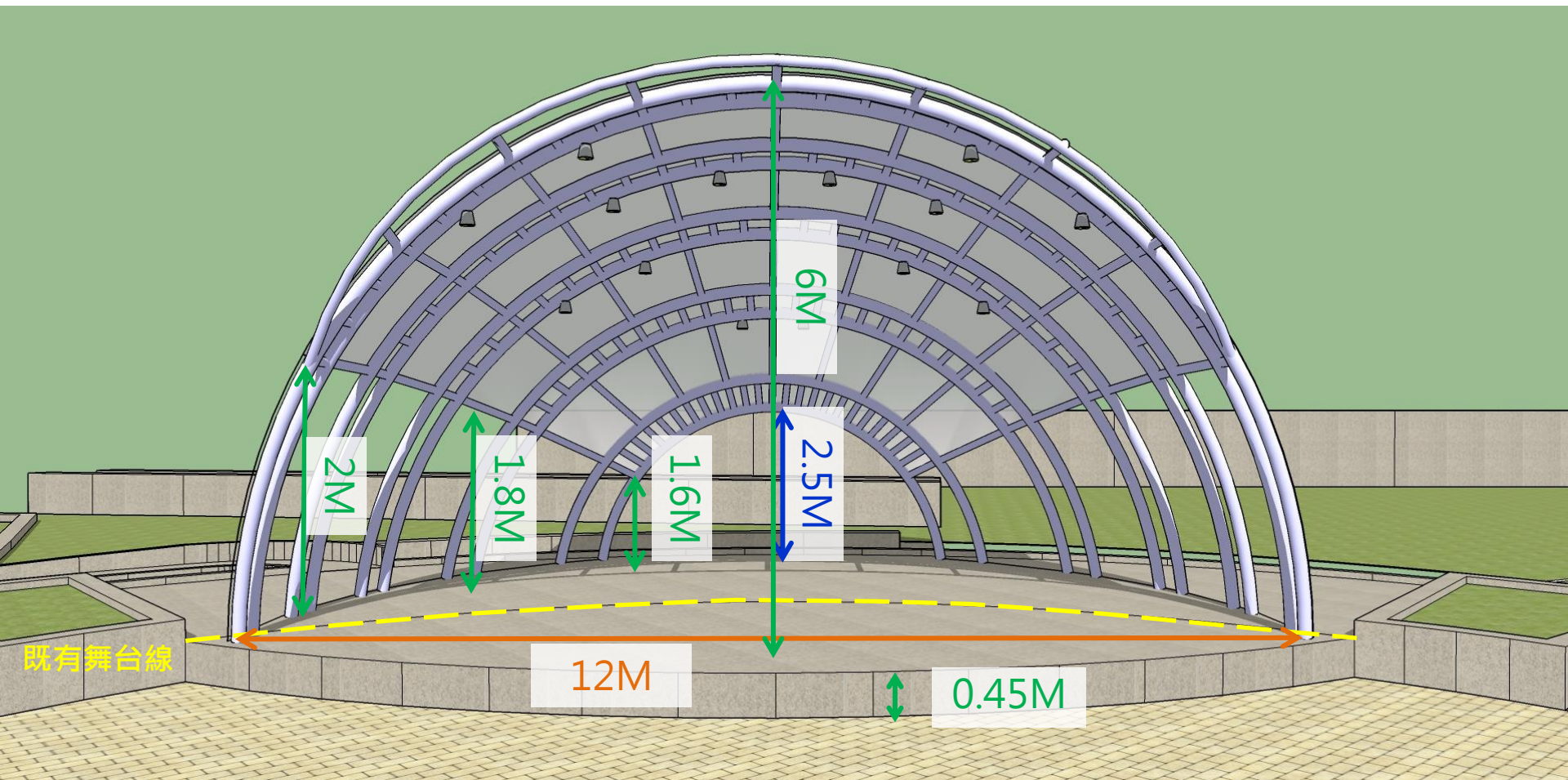
遮雨棚3D圖
