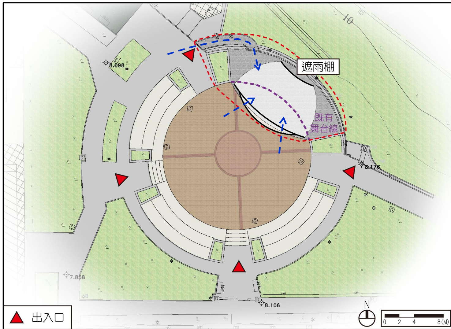
紫陽綠地舞台廣場平面圖
