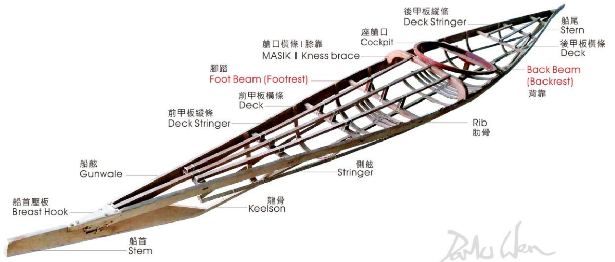
圖三、獨木舟結構圖
