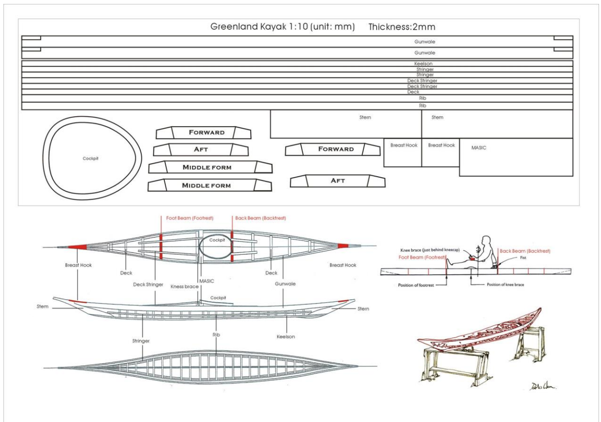
圖二、獨木舟骨架設計圖
