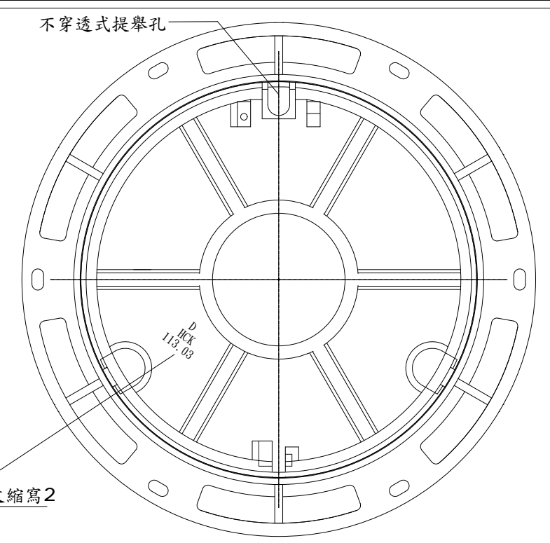
面蓋背面圖
