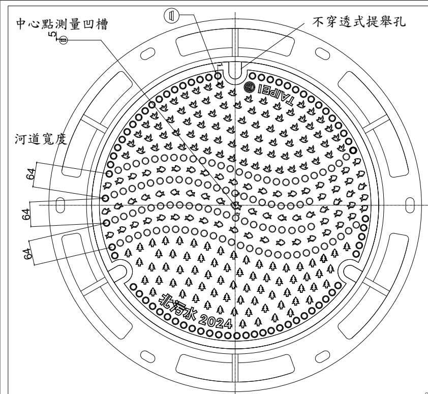
面蓋正面圖
