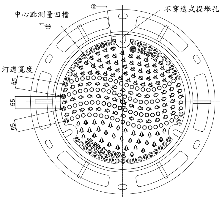
面蓋正面圖
