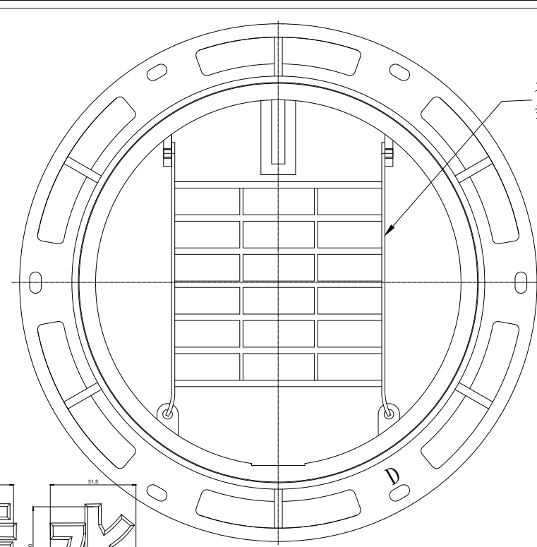
框座平面圖
