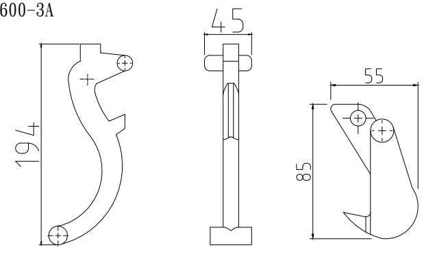
框蓋連結扣件示意圖 NTS 卡榫示意圖 NTS
