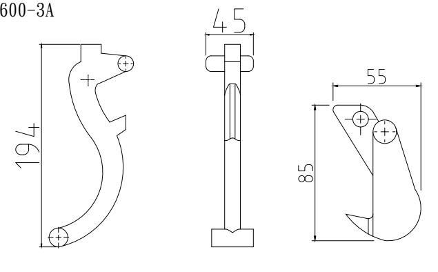
框蓋連結扣件示意圖 NTS 卡榫示意圖 NTS
