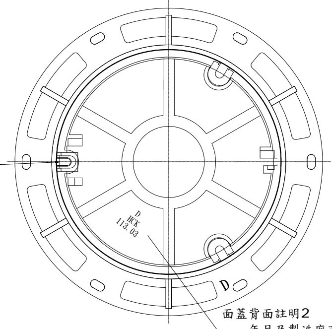
面蓋背面圖
