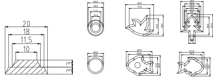
面蓋正面圖
