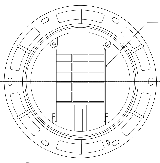
框座平面圖
