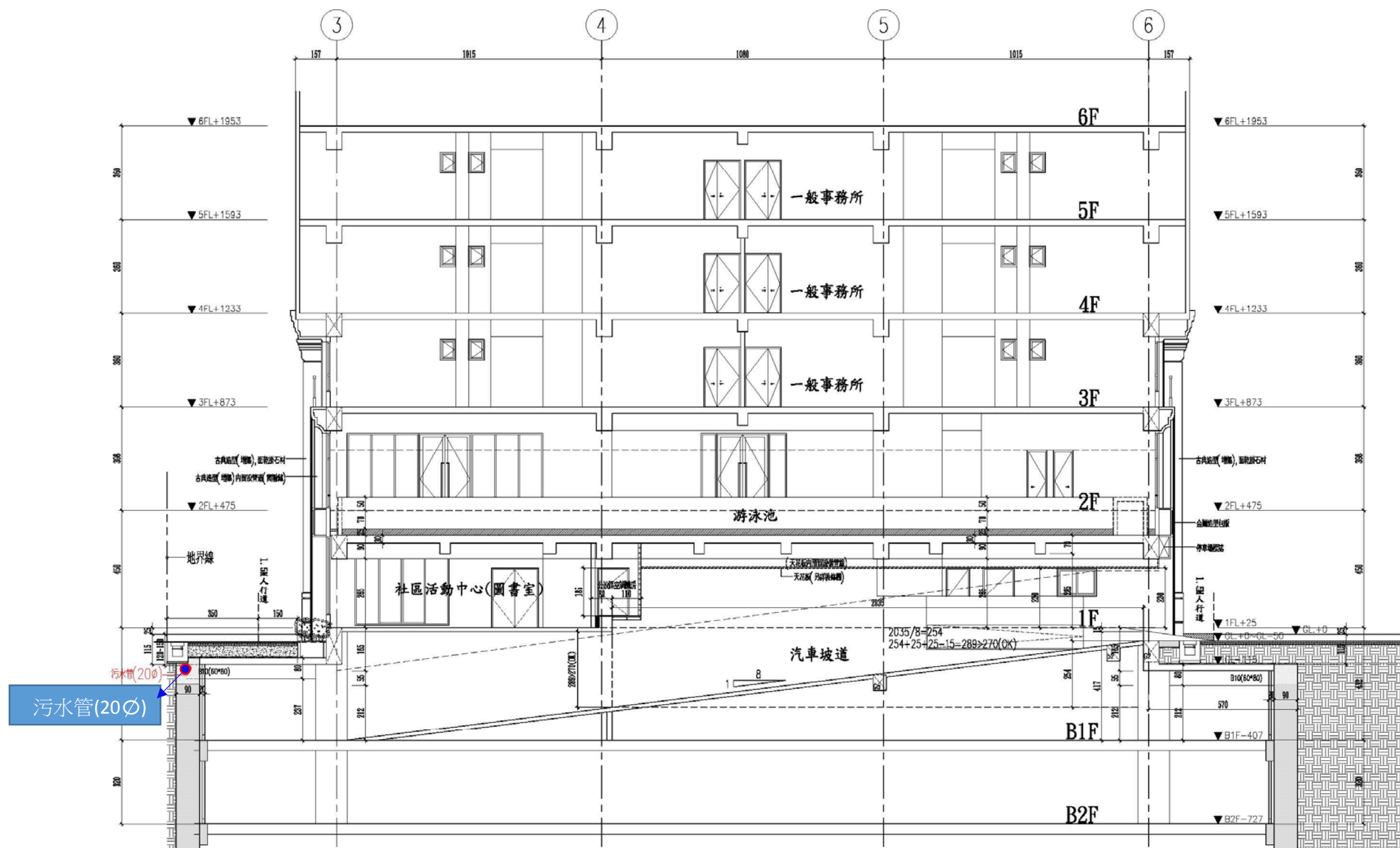
A-A牆剖面
