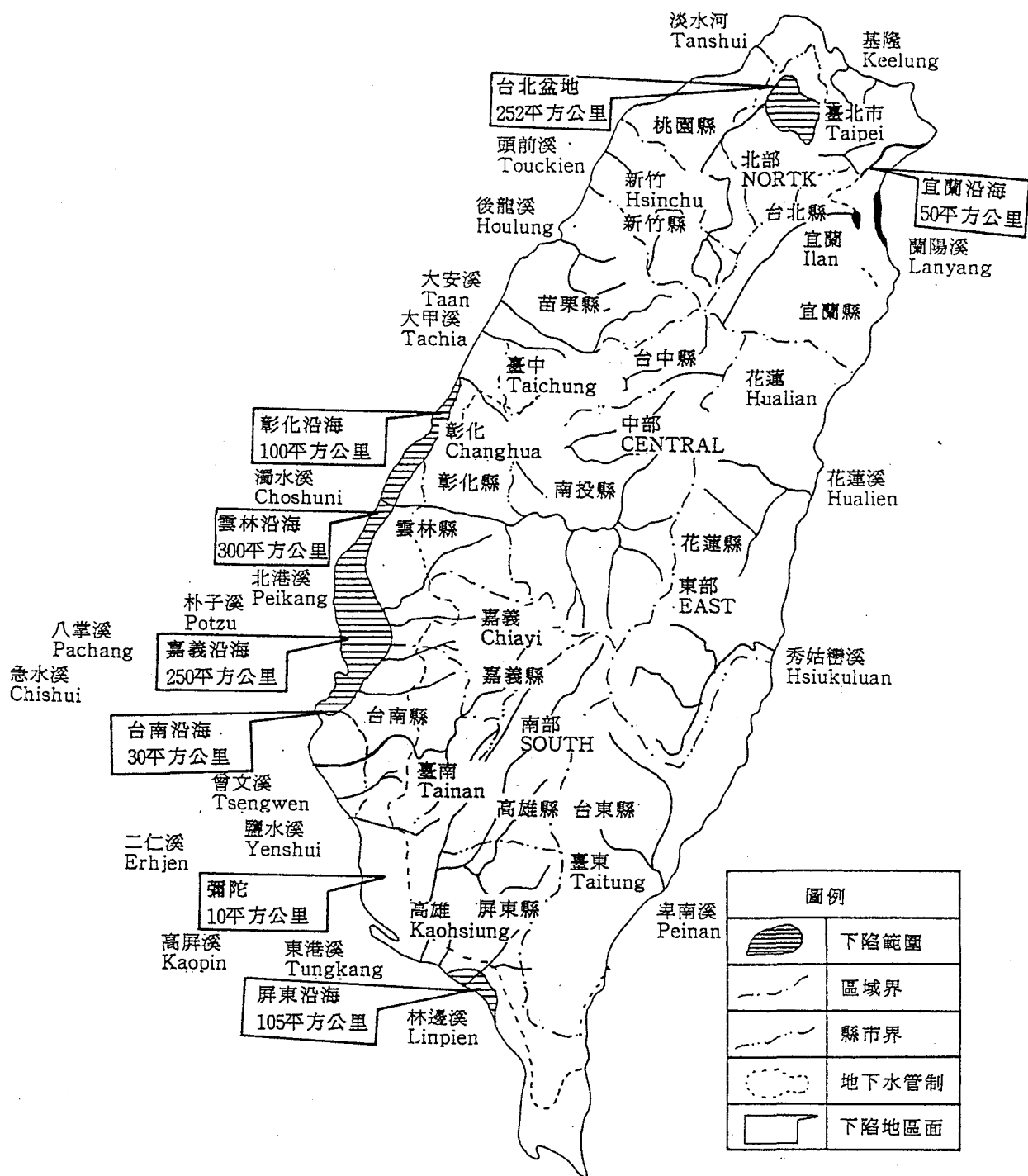
台灣地區地下水管制區暨地層下陷位置圖
