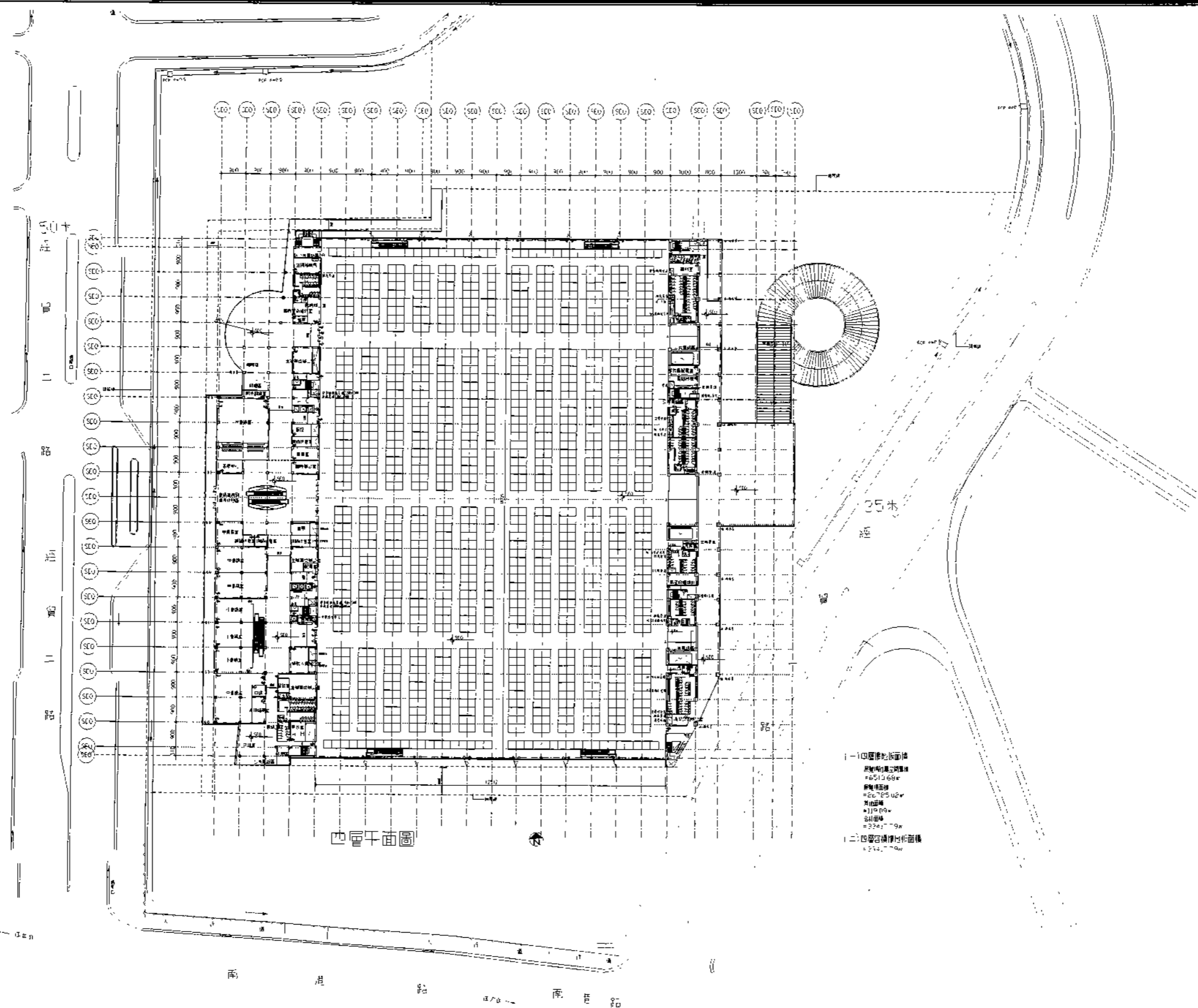
附圖 3-4 四層平面圖
