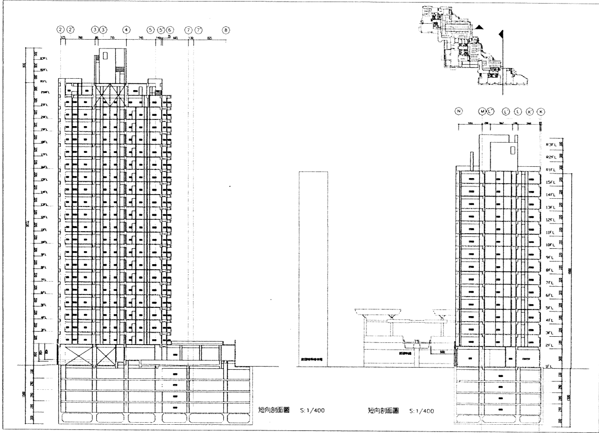
附圖3-10 短向剖面圖
