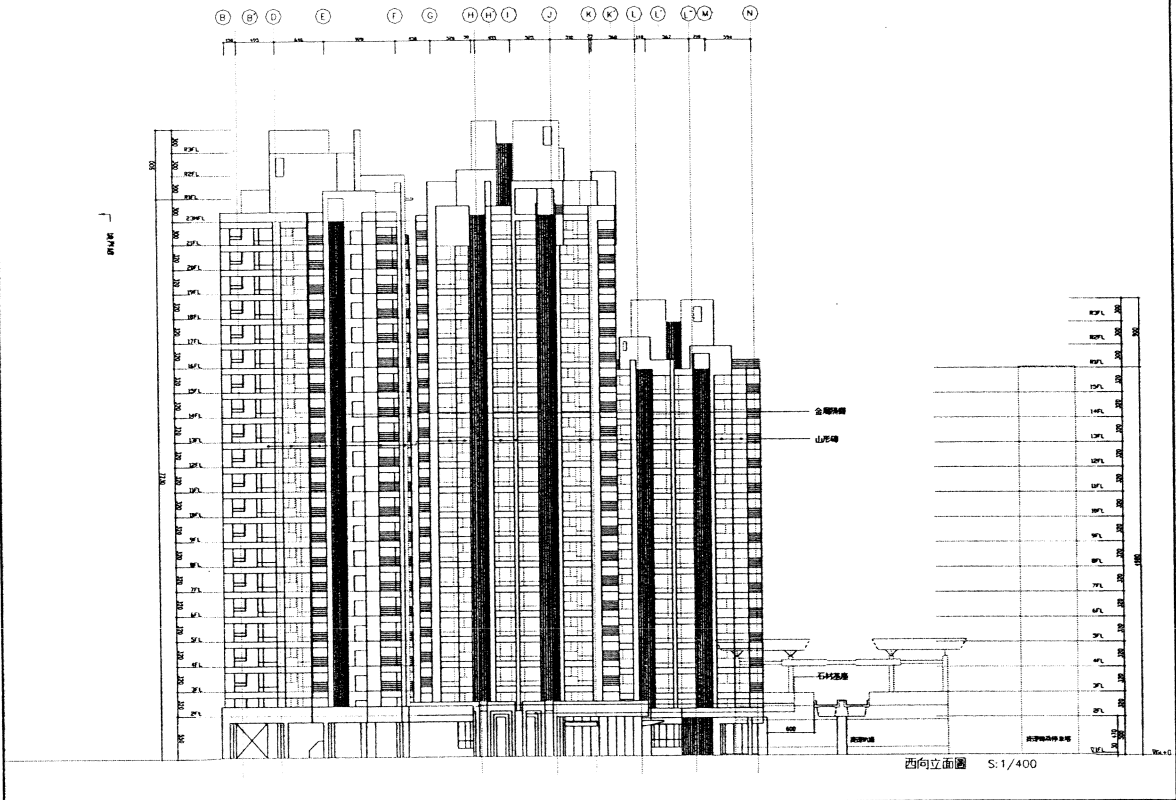
附圖3-8 西向立面圖
