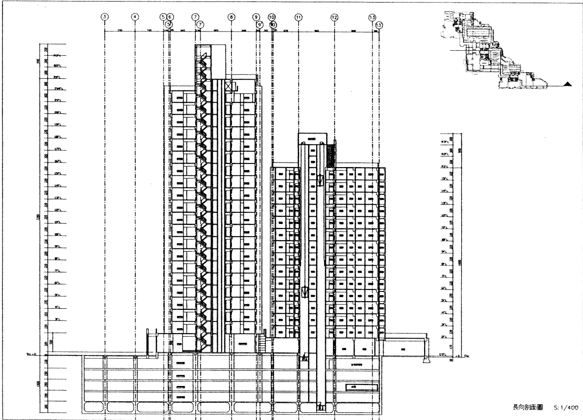
附圖3-9 長向剖面圖
