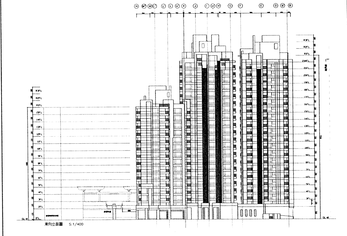
附圖3-7 東向立面圖
