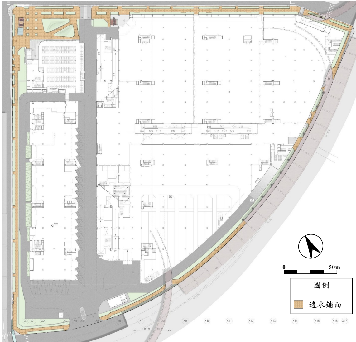
附圖 10-1 透水鋪面配置示意圖
