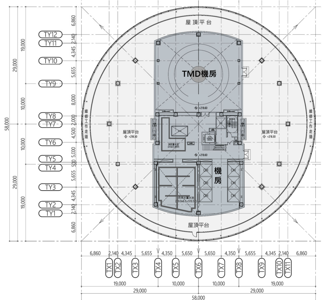
㊟ 屋突一層層平面圖 比例:1/400
