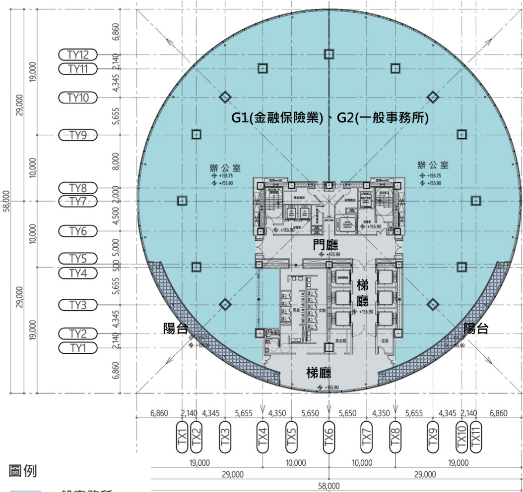
㊟ 三十一~四十三層平面圖 比例:1/400
