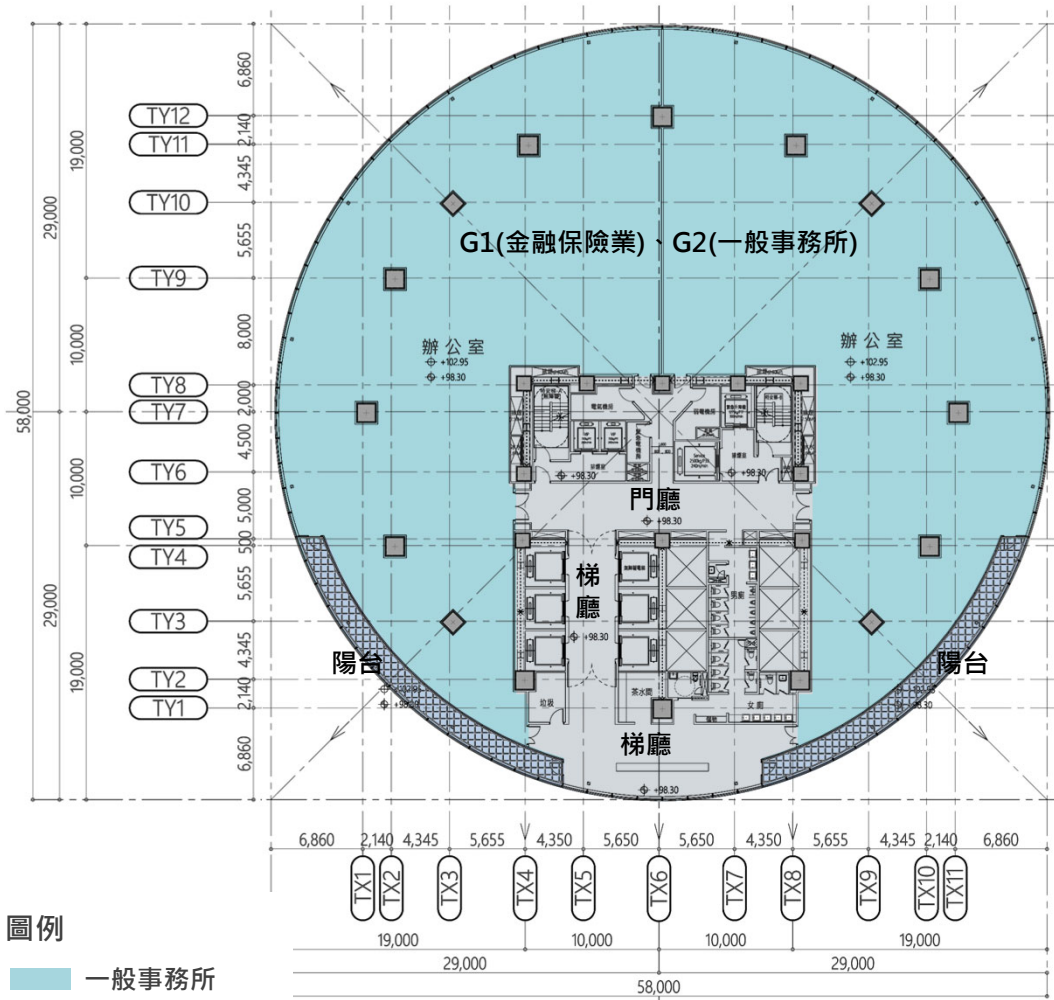
Ⓐ 十九層~二十五層平面圖 比例:1/400
