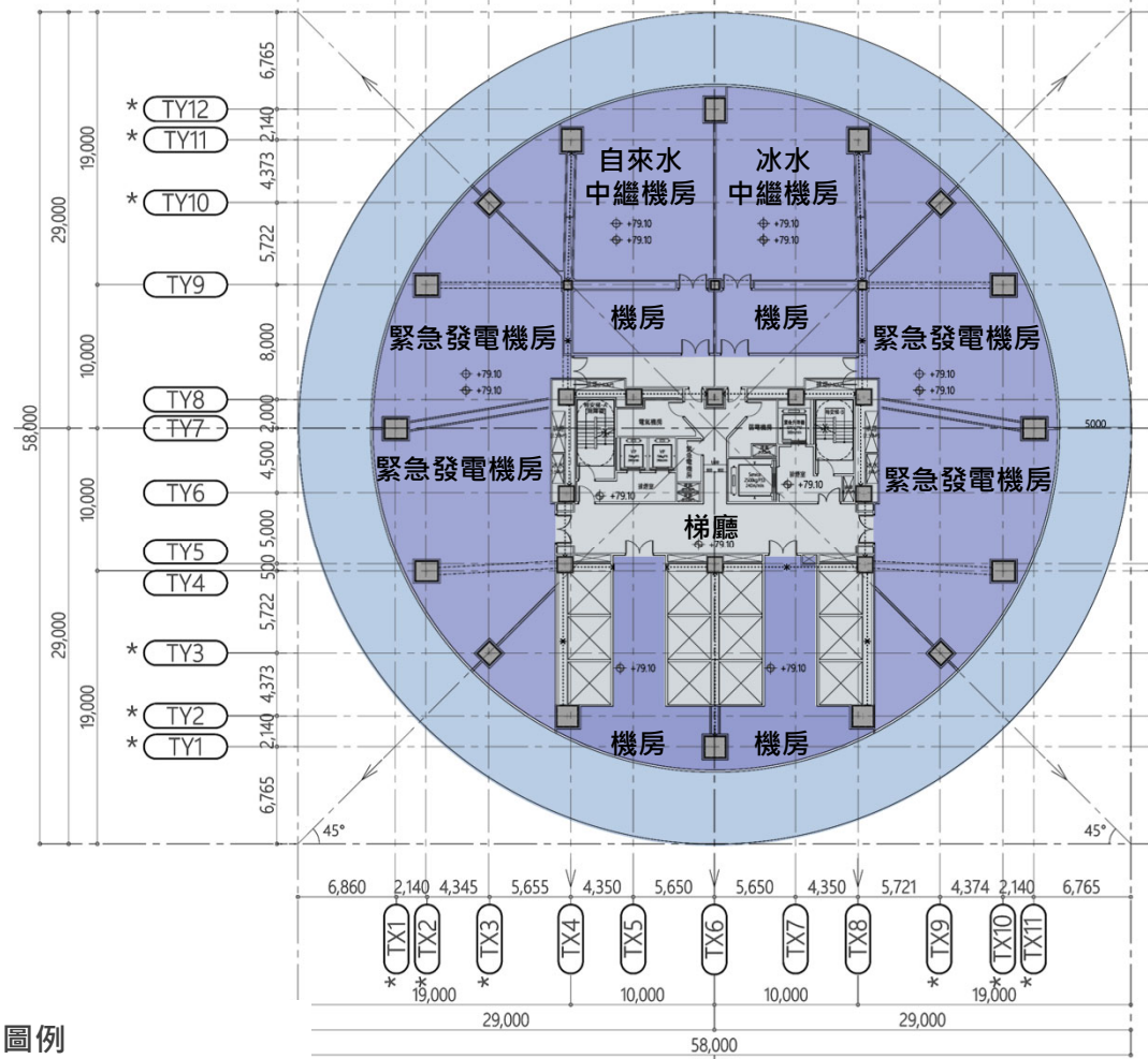
Ⓐ 十五層平面圖 比例:1/400
