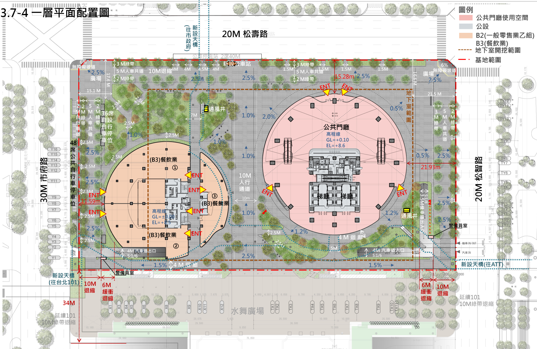
一層平面配置圖 比例:1/600
