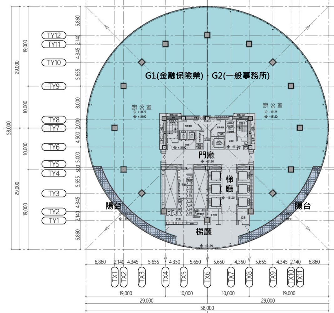
Ⓐ 二十六層~二十八層平面圖 比例:1/400
