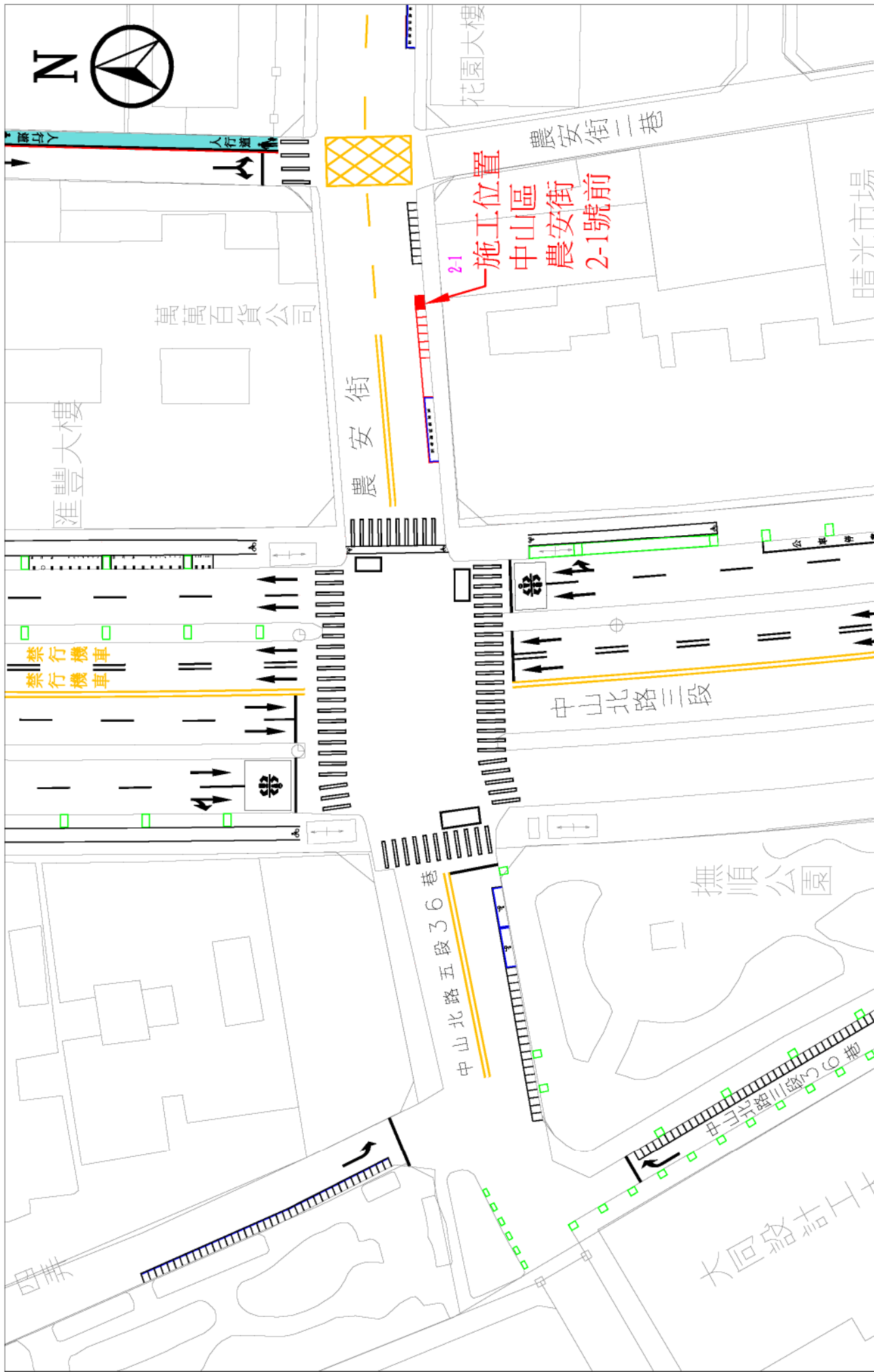
施工位置圖:中山區農安街2之1號前
