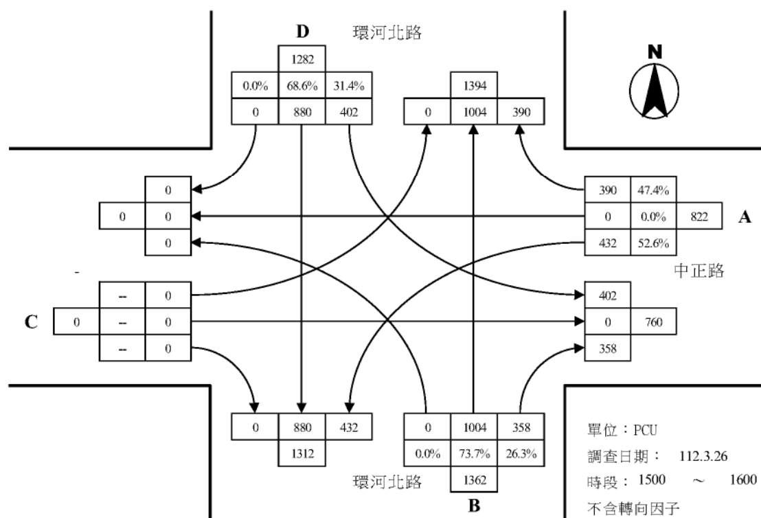
環河北路與中正路路口假日離峰轉向交通量示意圖
