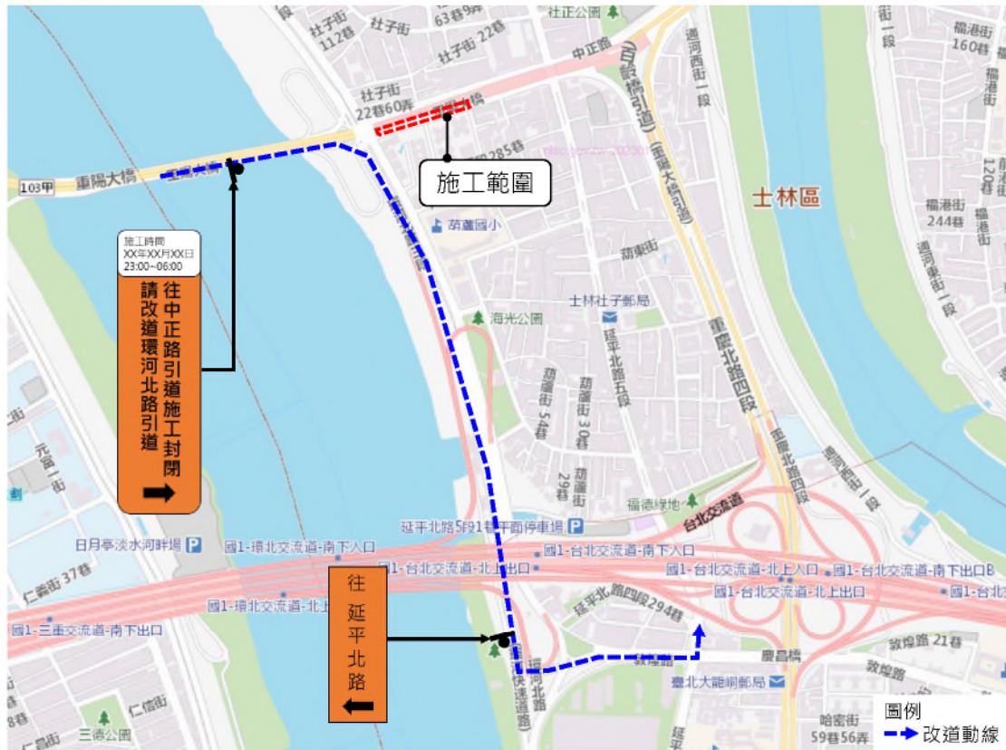
圖 4.2-3 封閉重陽橋往東方向銜接中正路引道改道動線圖
