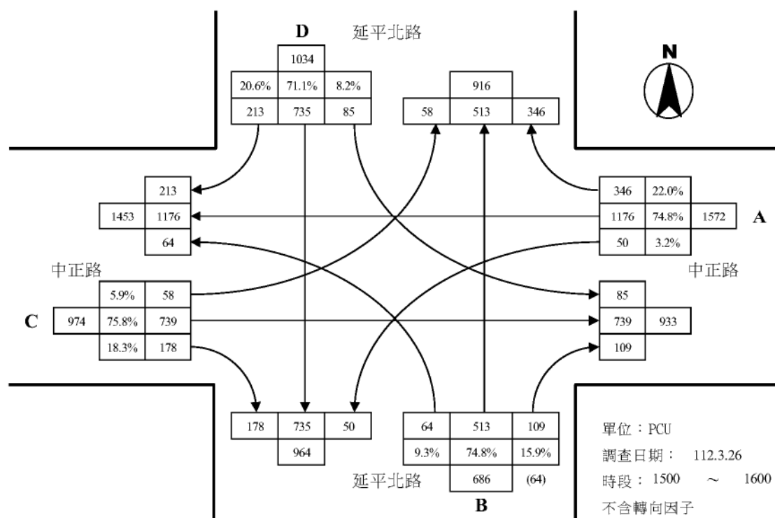
延平北路與中正路路口假日離峰轉向交通量示意圖
