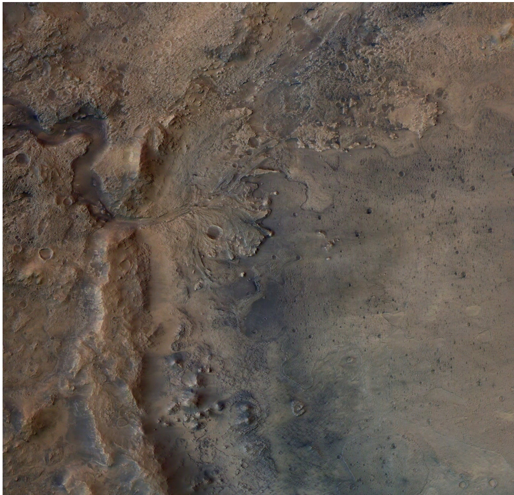
↑圖2. 傑澤羅隕石坑。在圖中可以明顯的看到隕石坑中古老的河道與三角洲。
