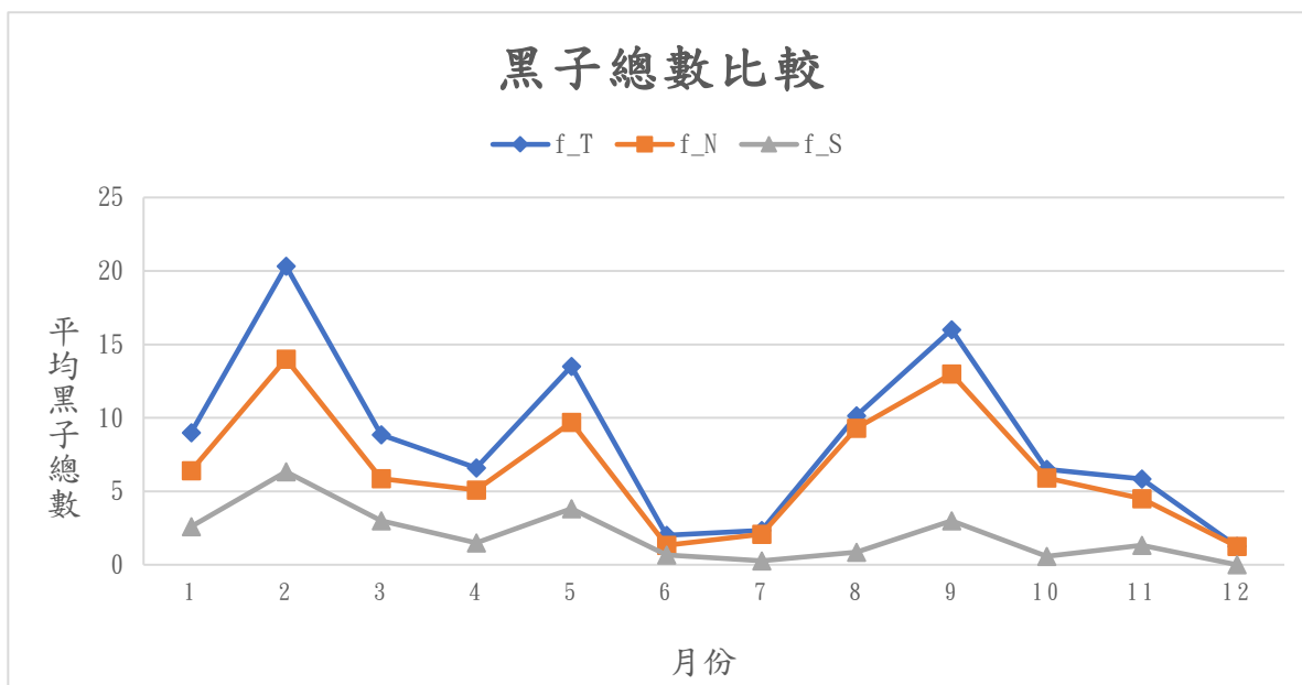
本圖為2016年各月的平均黑子總數變化圖，其中f_T代表整個太陽可見半球面的黑子總數，f_N與f_S則分別代表可見半球面中之北半球與南半球的黑子總數。
