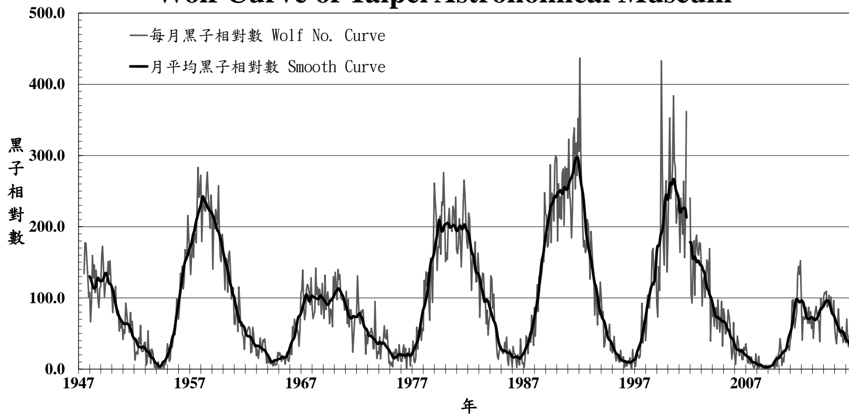
本圖為臺北天文館自1947年7月至2016年12月的每月黑子相對數（灰色細線）與月平均黑子相對數（黑色粗線）曲線圖。兩曲線均尚未做K值的修正。
