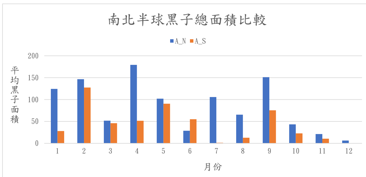
本圖為2016年各月的南北半球黑子總面積變化圖，其中A_N與A_S分別代表可見半球面中之北半球與南半球的黑子總面積。面積以「太陽半球面總面積的百萬分之一」為單位，此為太陽投影觀測的慣用單位。
