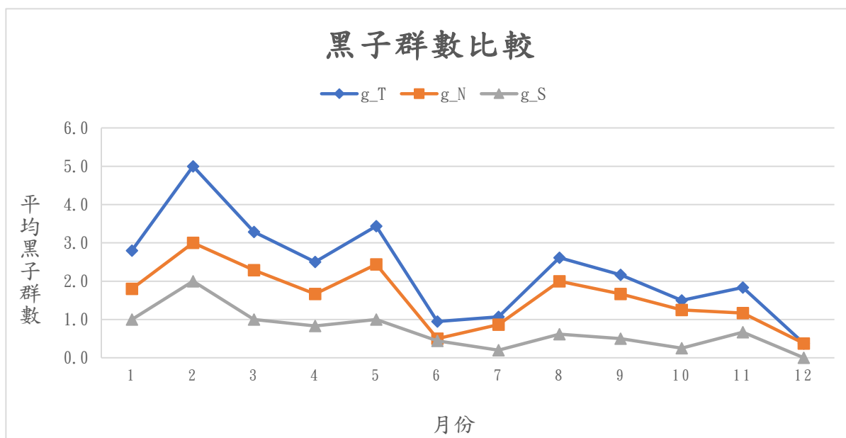
本圖為2016年各月的平均黑子群數變化圖，其中g_T代表整個太陽可見半球面的黑子群數，g_N與g_S則分別代表可見半球面中之北半球與南半球的黑子群數。
