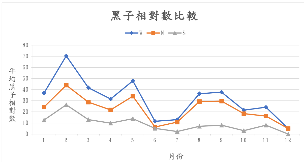
本圖為2016年各月的平均黑子相對數變化圖，其中W代表整個太陽可見半球面的黑子相對數，N與S則分別代表可見半球面中之北半球與南半球的黑子相對數。
