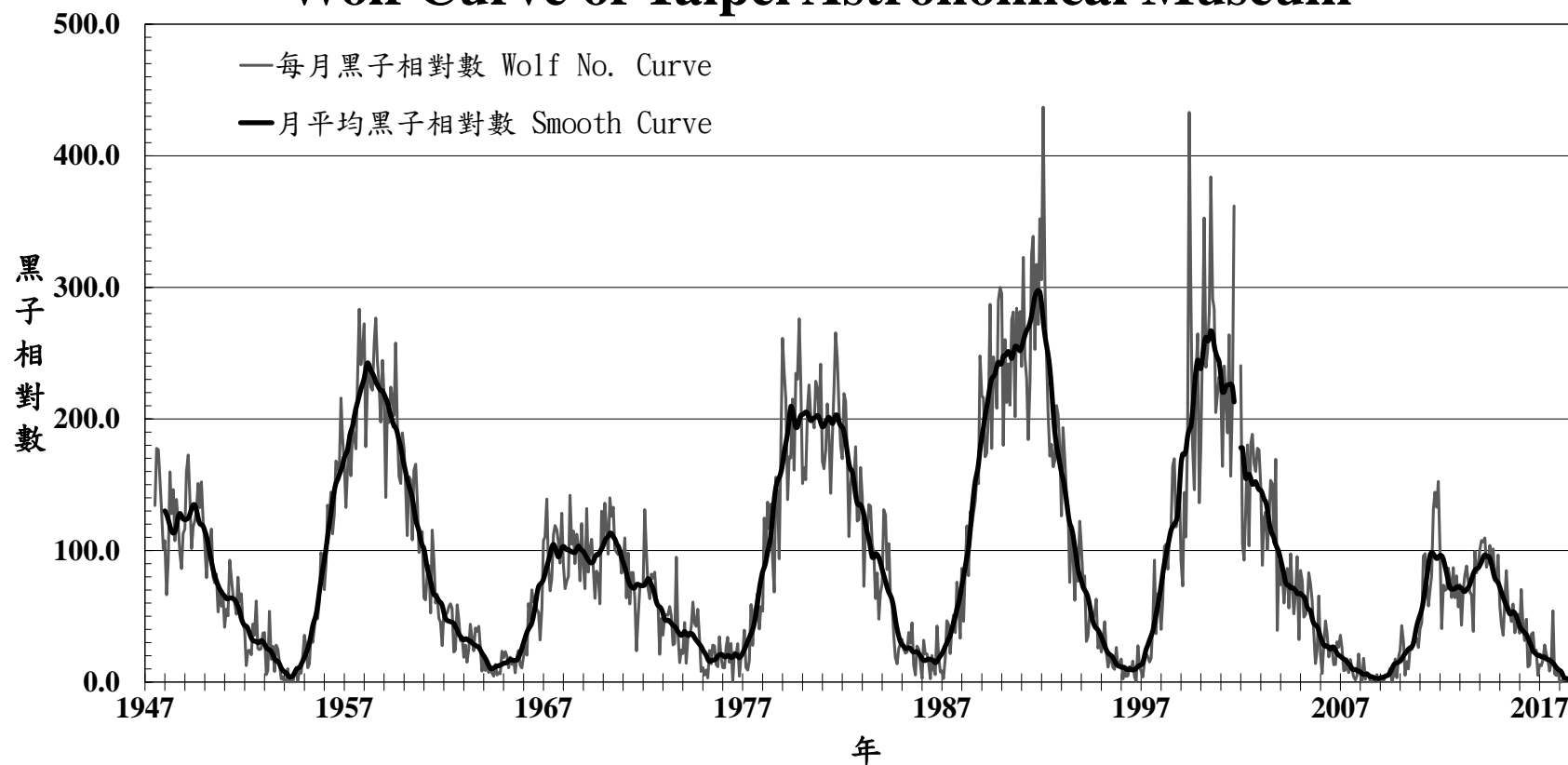
本圖為臺北天文館自1947年7月至2018年12月的每月黑子相對數（灰色細線）與月平均黑子相對數（黑色粗線）曲線圖。兩曲線均尚未做K值的修正。
