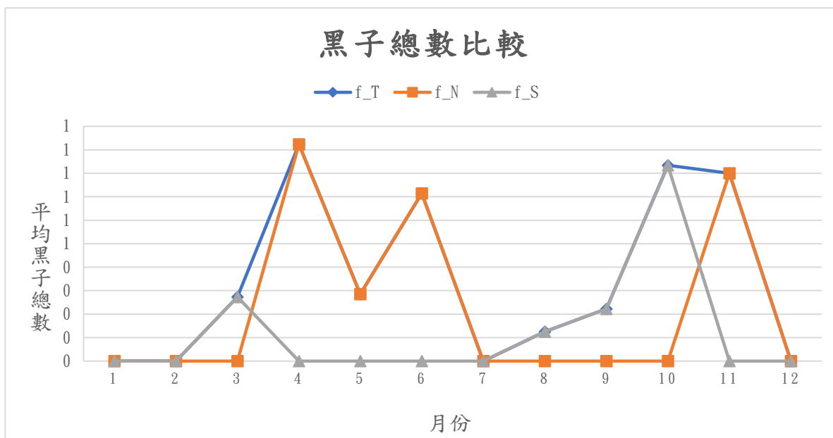
本圖為2018年各月的平均黑子總數變化圖，其中f_T代表整個太陽可見半球面的黑子總數，f_N與f_S則分別代表可見半球面中之北半球與南半球的黑子總數。
