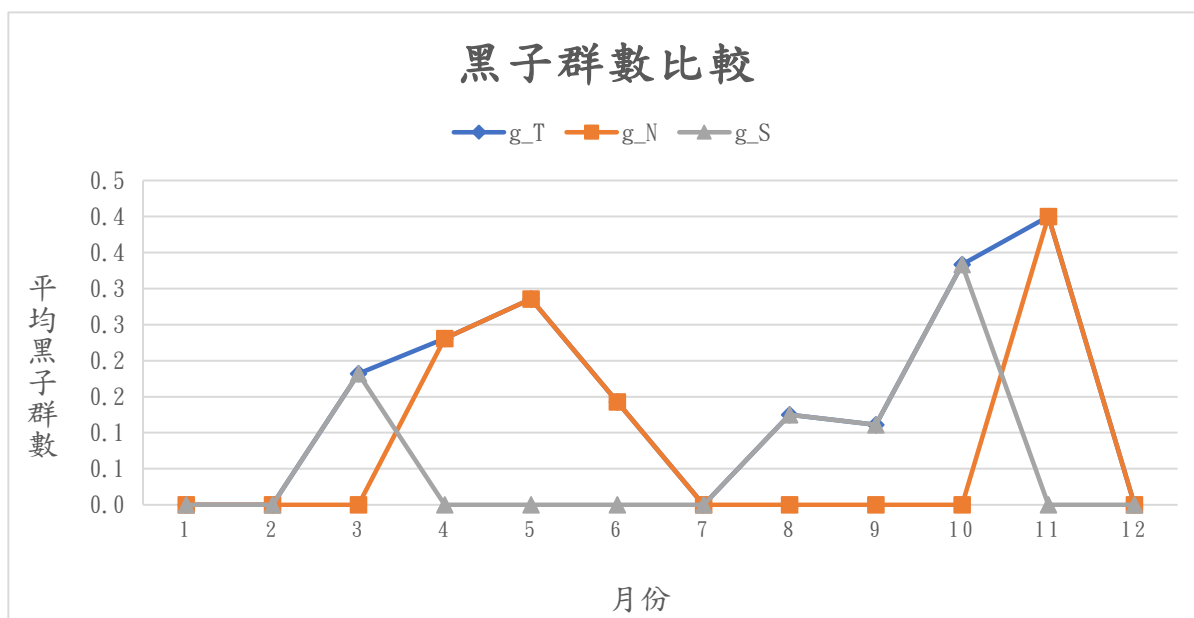
本圖為2018年各月的平均黑子群數變化圖，其中g_T代表整個太陽可見半球面的黑子群數，g_N與g_S則分別代表可見半球面中之北半球與南半球的黑子群數。
