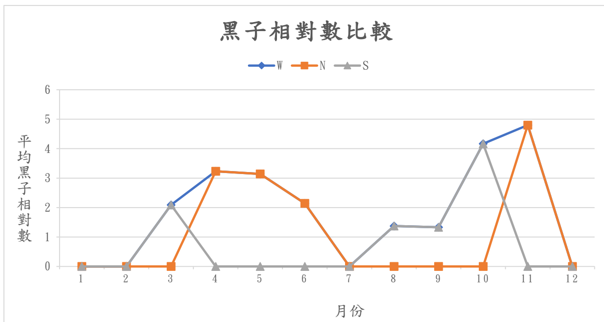
本圖為2018年各月的平均黑子相對數變化圖，其中W代表整個太陽可見半球面的黑子相對數，N與S則分別代表可見半球面中之北半球與南半球的黑子相對數。
