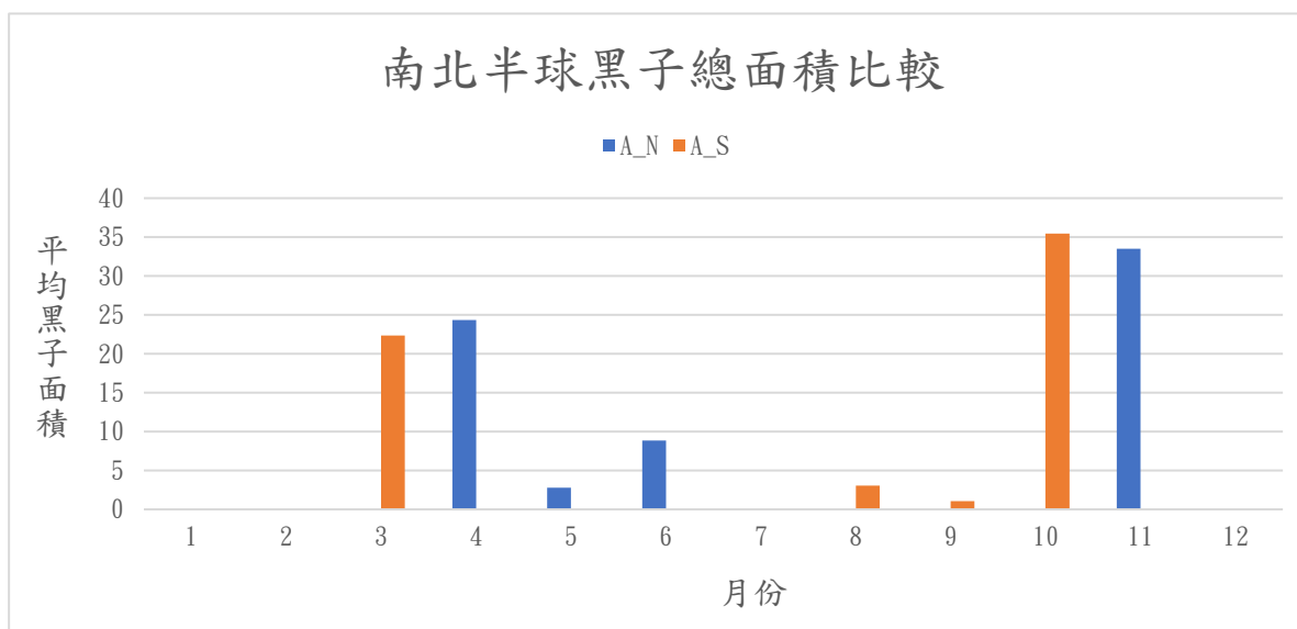
本圖為2018年各月的南北半球黑子總面積變化圖，其中A_N與A_S分別代表可見半球面中之北半球與南半球的黑子總面積。面積以「太陽半球面總面積的百萬分之一」為單位，此為太陽投影觀測的慣用單位。
