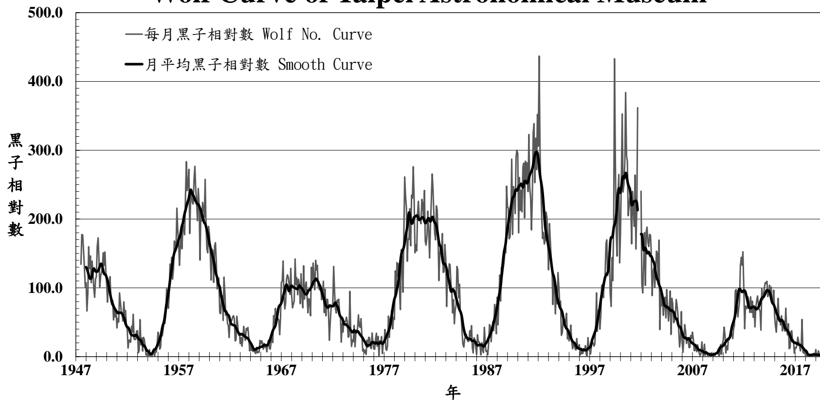
本圖為臺北天文館自1947年7月至2019年12月的每月黑子相對數（灰色細線）與月平均黑子相對數（黑色粗線）曲線圖。兩曲線均尚未做K值的修正。
