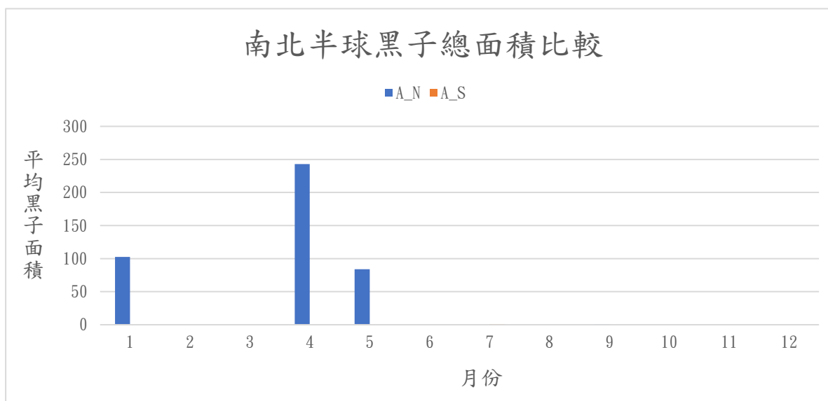
本圖為2019年各月的南北半球黑子總面積變化圖，其中A_N與A_S分別代表可見半球面中之北半球與南半球的黑子總面積。面積以「太陽半球面總面積的百萬分之一」為單位，此為太陽投影觀測的慣用單位。
