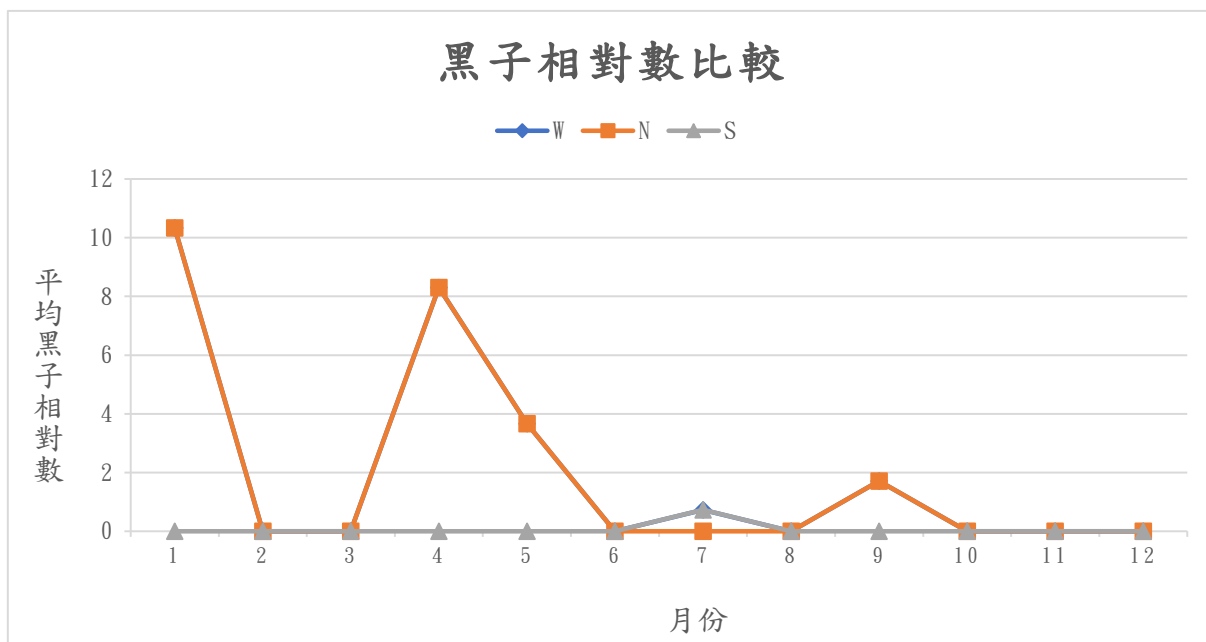
本圖為2019年各月的平均黑子相對數變化圖，其中W代表整個太陽可見半球面的黑子相對數，N與S則分別代表可見半球面中之北半球與南半球的黑子相對數。
