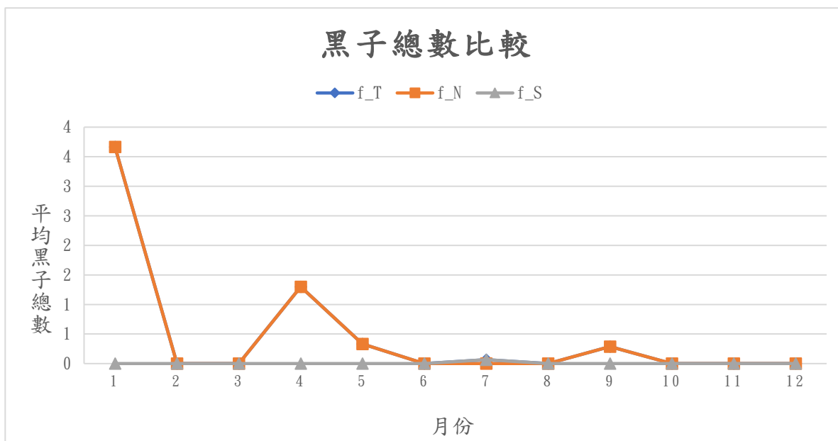
本圖為2019年各月的平均黑子總數變化圖，其中f_T代表整個太陽可見半球面的黑子總數，f_N與f_S則分別代表可見半球面中之北半球與南半球的黑子總數。
