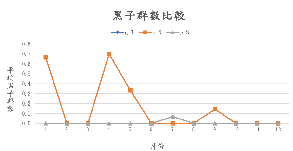
本圖為2019年各月的平均黑子群數變化圖，其中g_T代表整個太陽可見半球面的黑子群數，g_N與g_S則分別代表可見半球面中之北半球與南半球的黑子群數。
