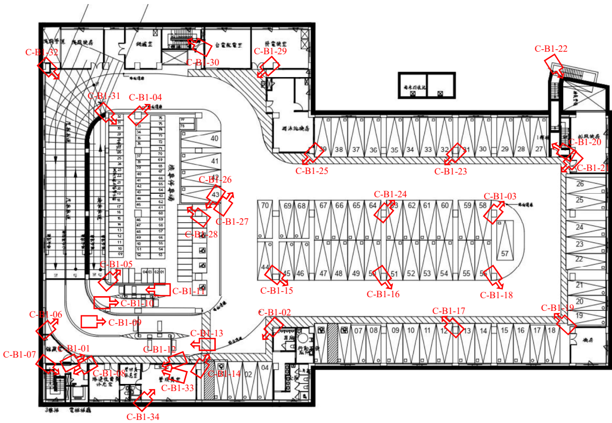
B1 平面圖
