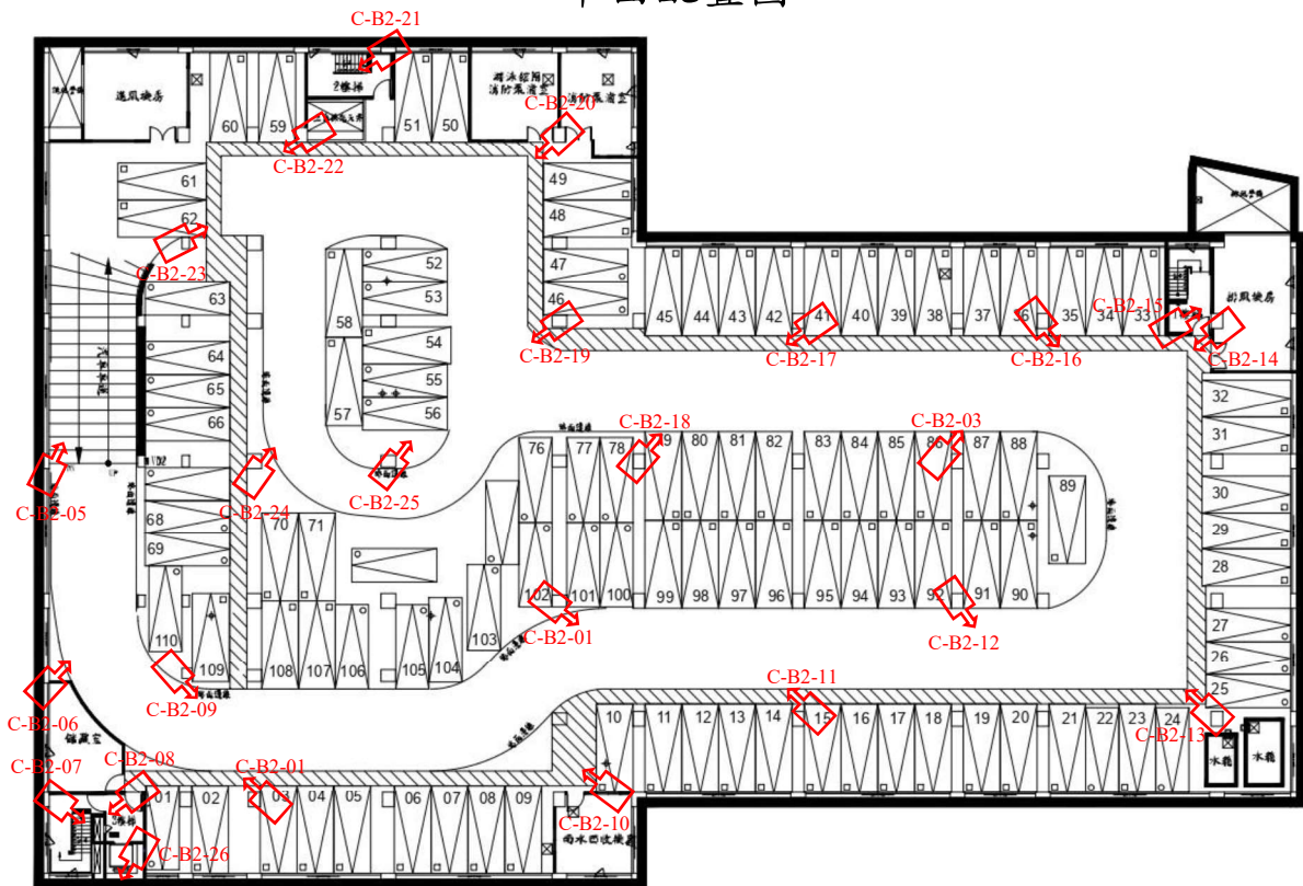
B2平面圖
