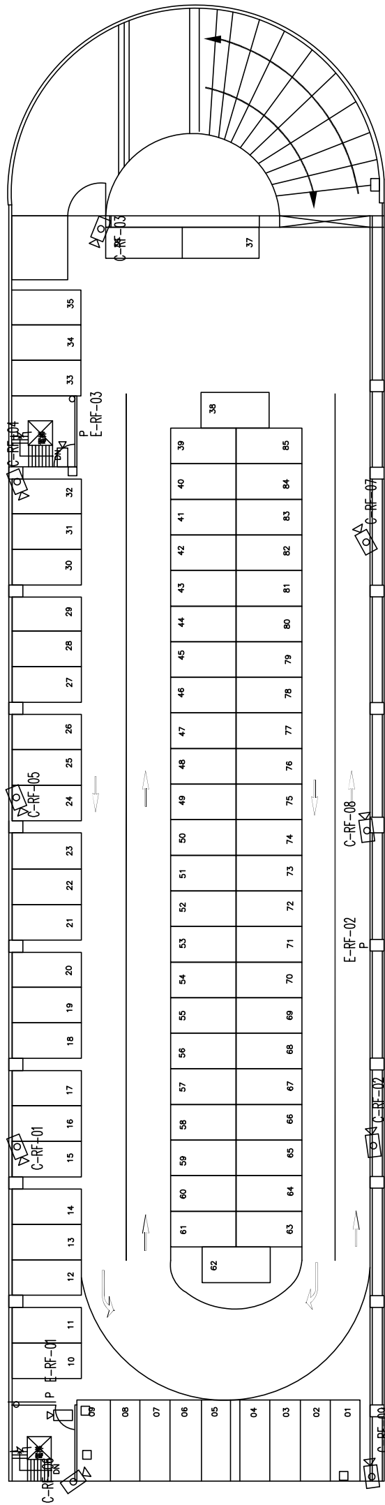
屋頂層平面圖
