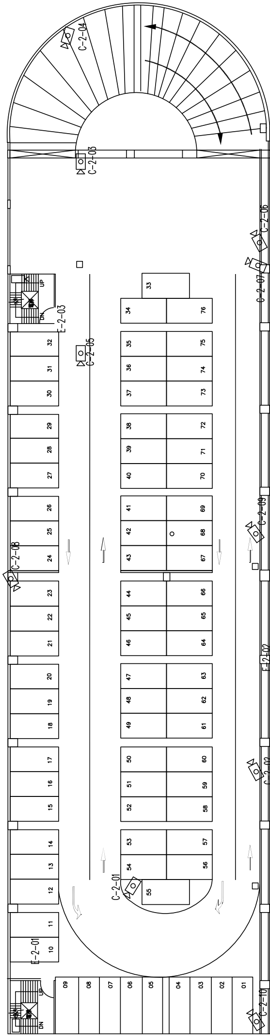
二層平面圖
