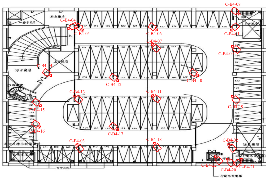
B4平面圖
