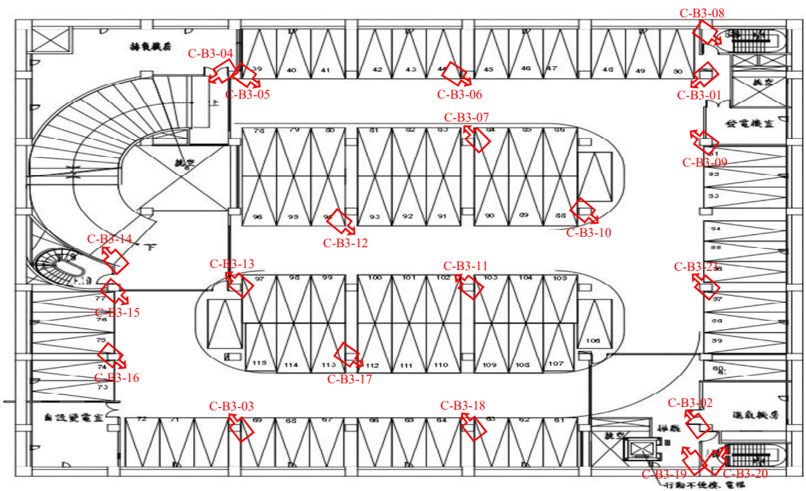
B3平面圖
