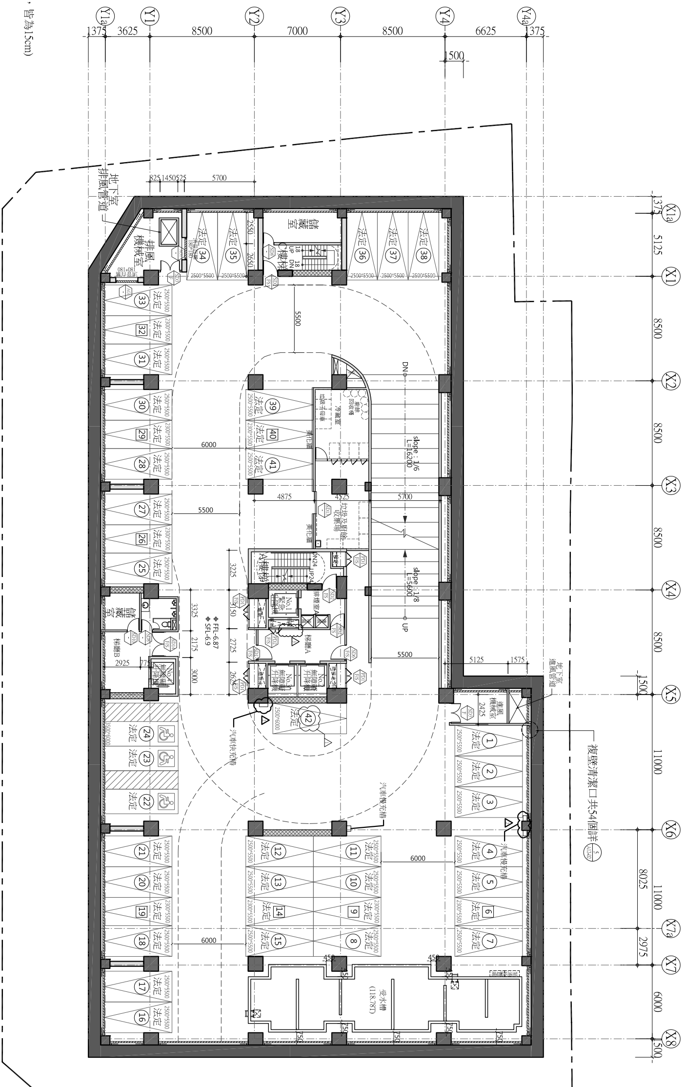
① 地下室二層平面圖 S:A1=1/150 S:A3=1/300
