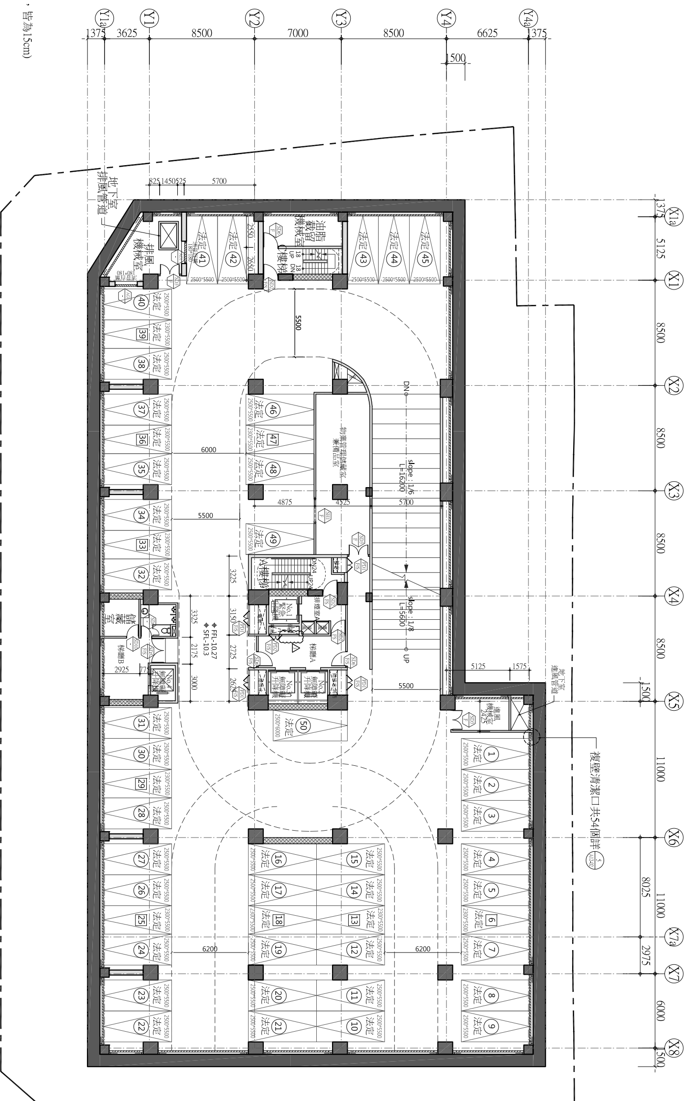
⊕ 地下三層平面圖 S:A1=1/150 S:A3=1/300
