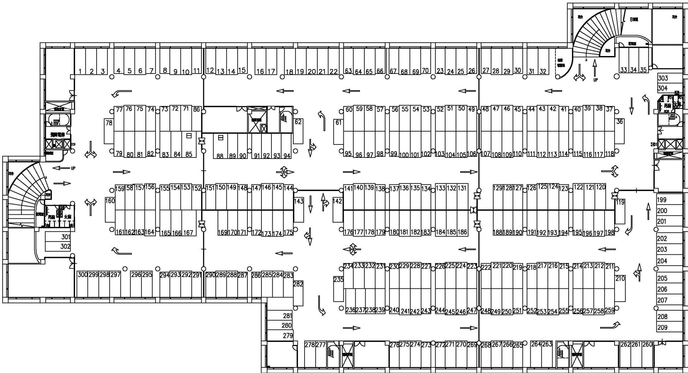
林森公園地下三層平面圖
