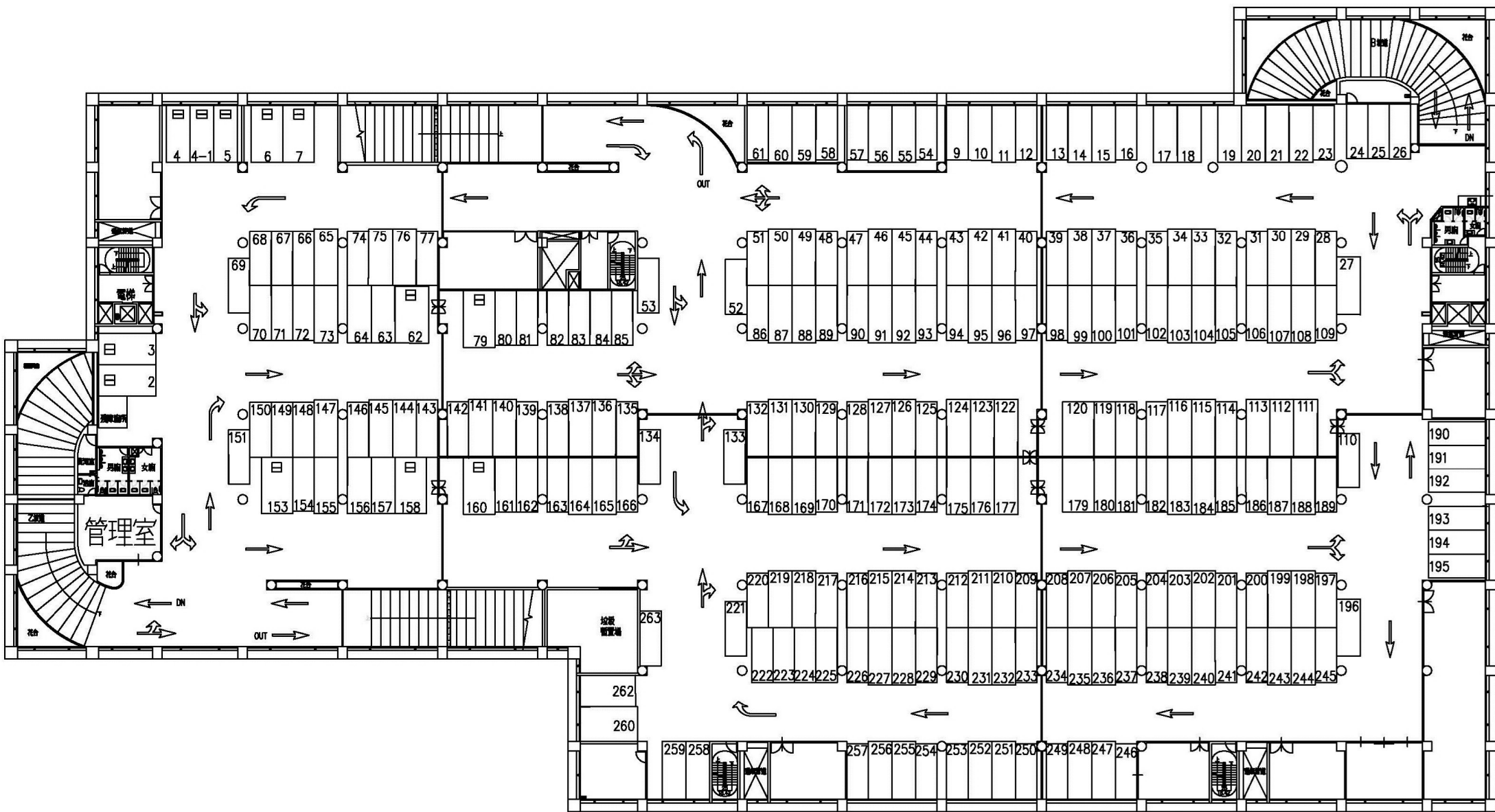
林森公園地下一層平面圖
