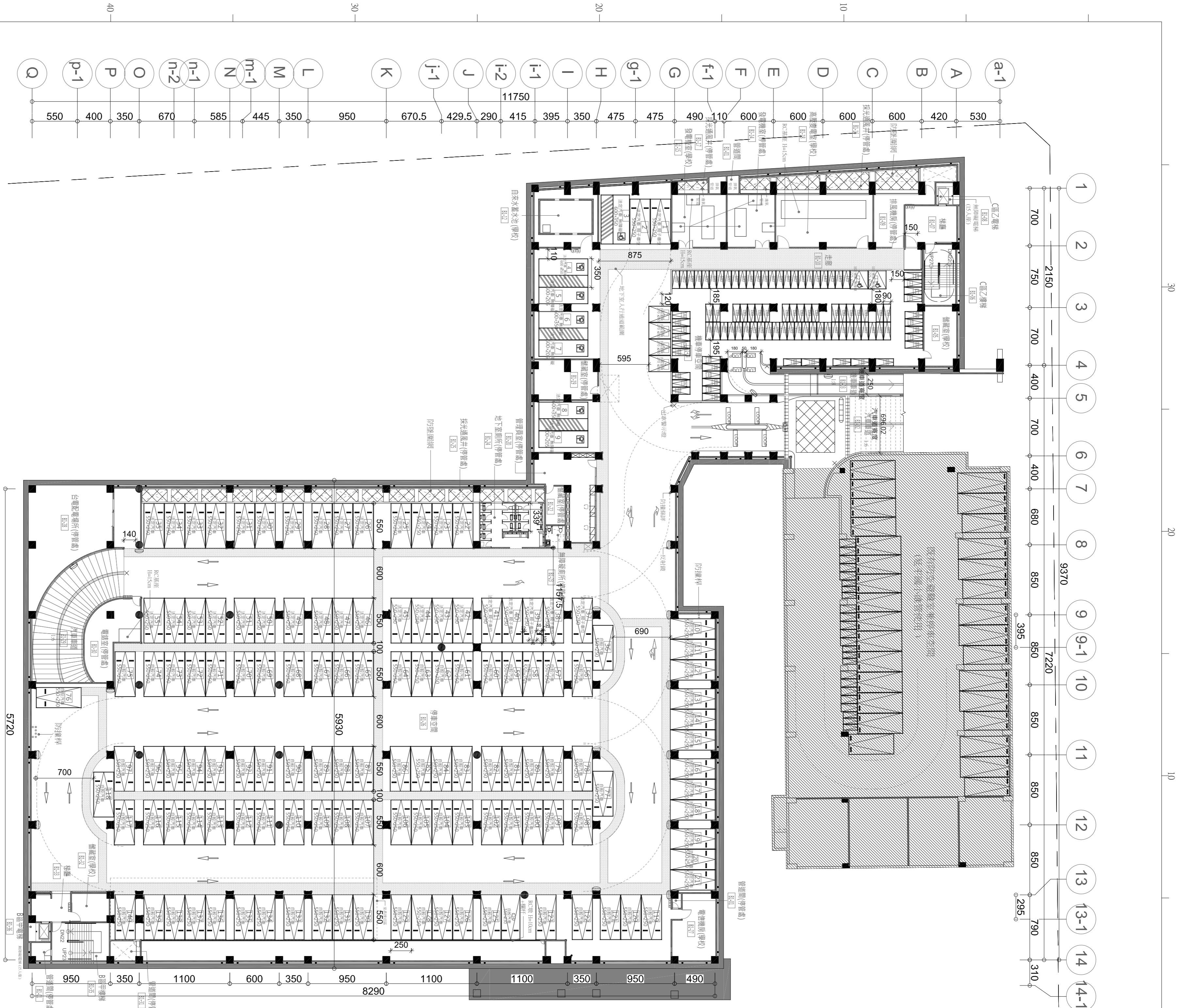
1 地下一層平面圖 A2-02 A1:1:300
