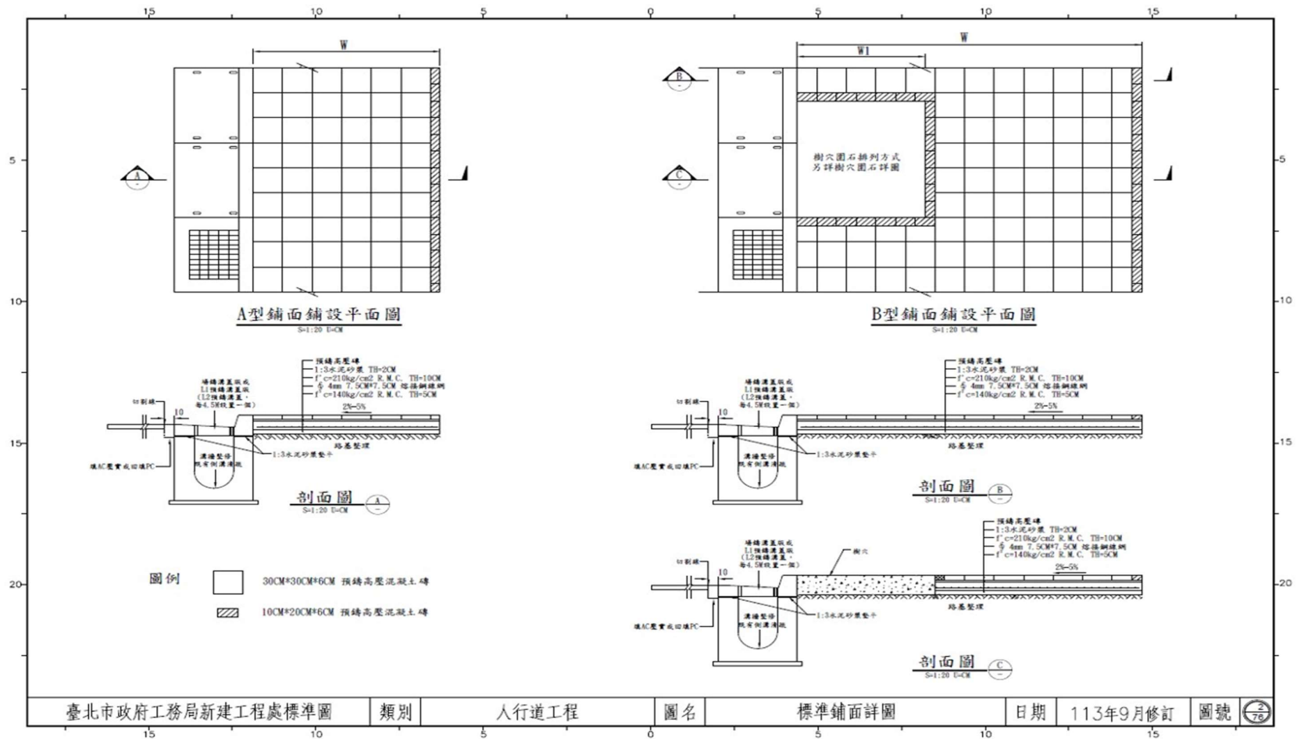
圖1 實體人行道標準圖
