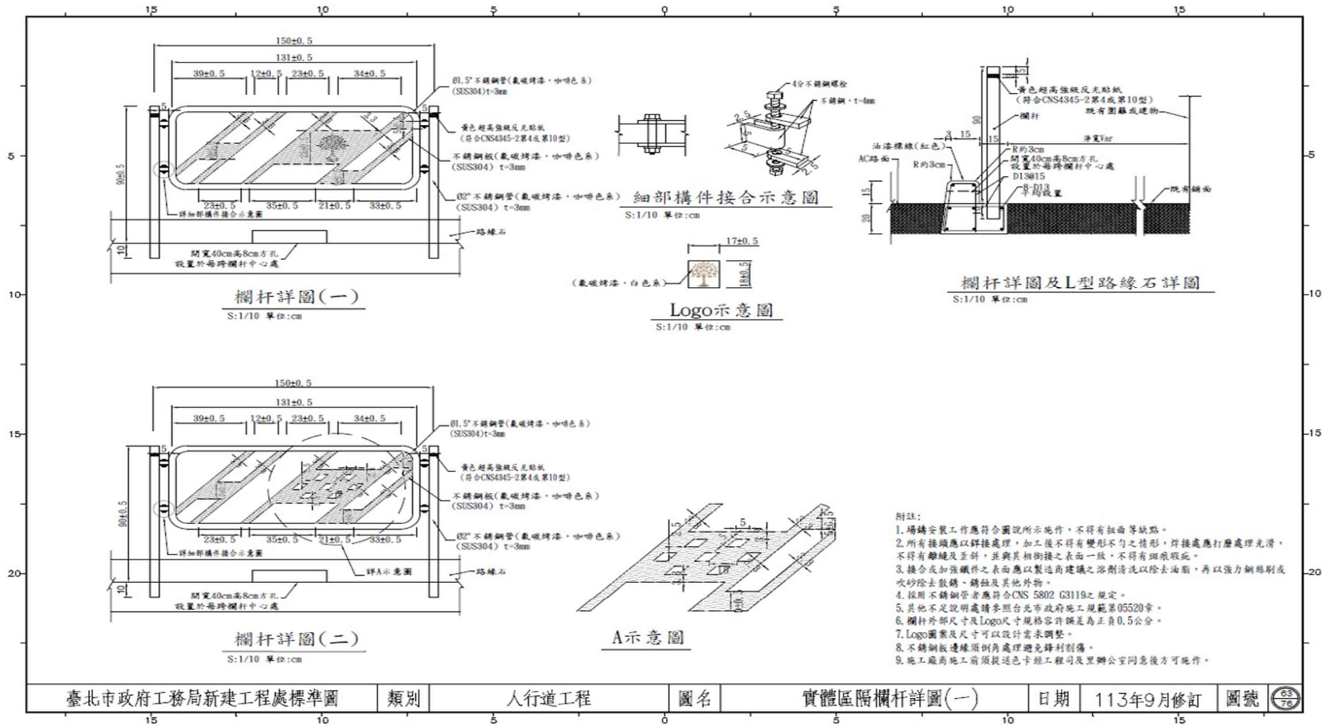
圖2 實體區隔標準圖
