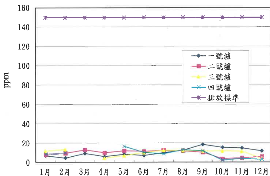
圖參之一(二)4 109 年一氧化碳(CO)排放監測值
