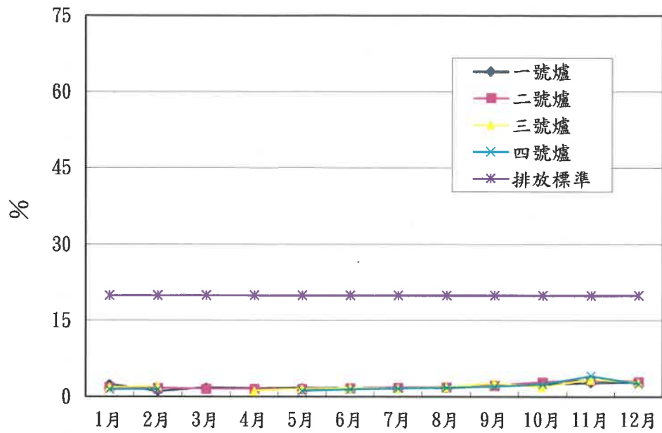
圖參之一(二)5 109 年不透光率排放監測值
