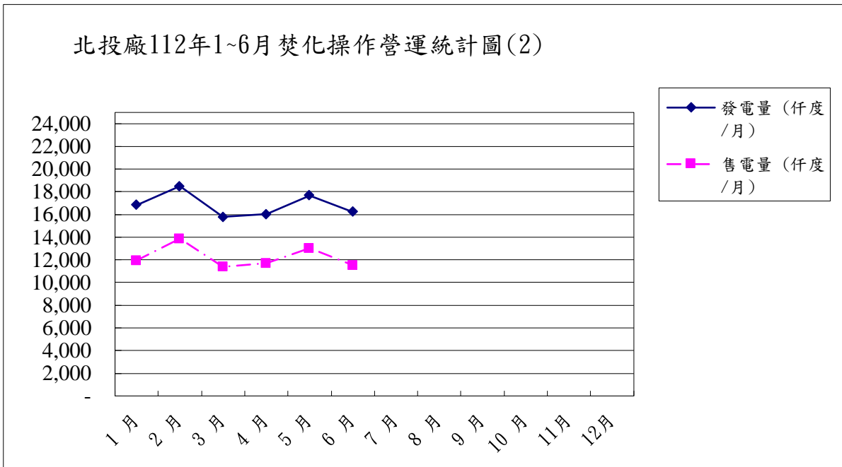
圖貳之一-2-112 年焚化操作營運統計圖
