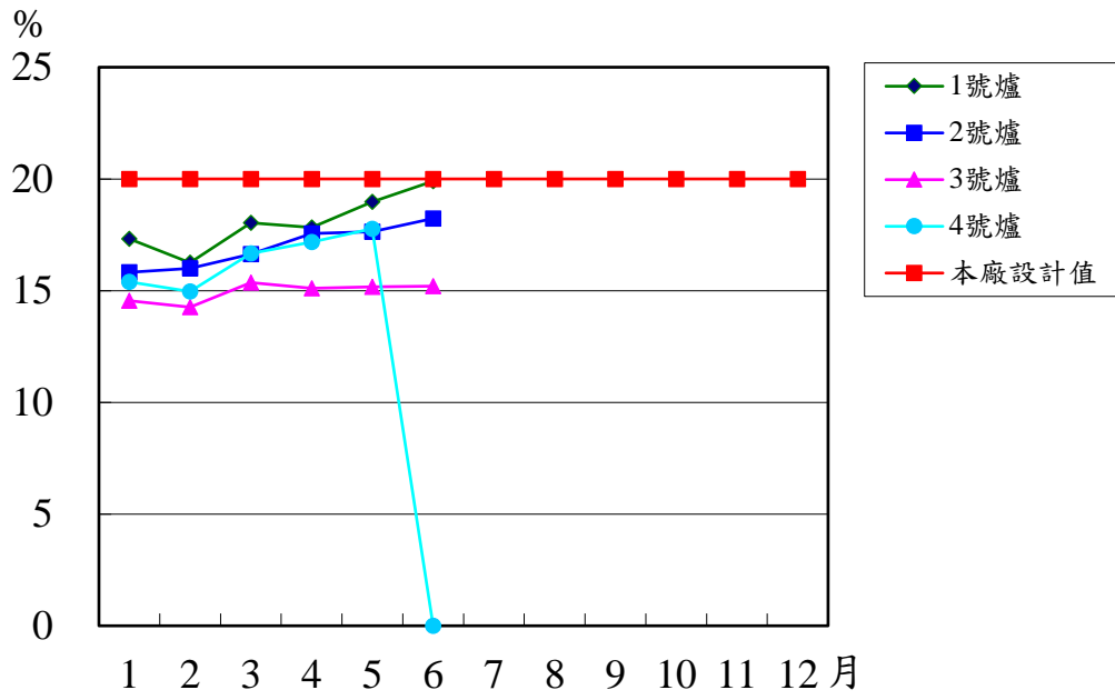
圖參之一(二)-7-113 年含水率排放監測值
