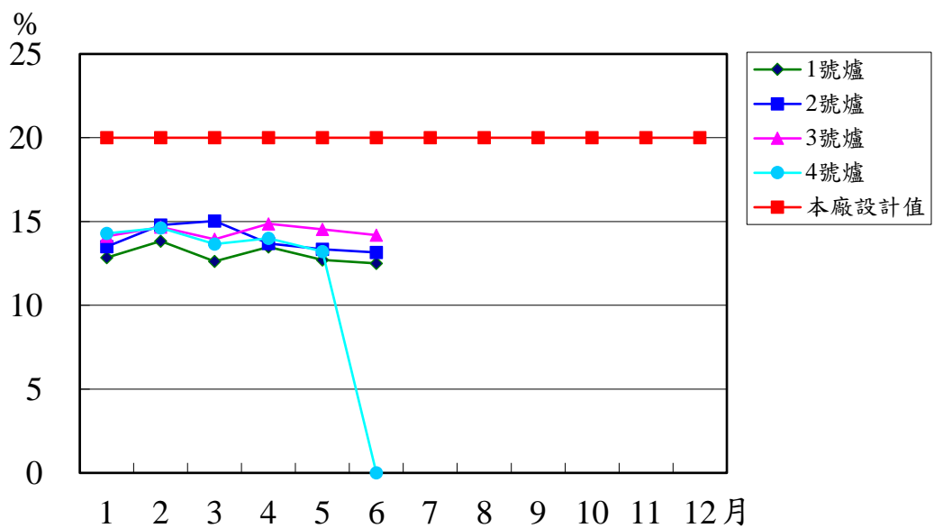
圖參之一(二)-6-113 年含氧率排放監測值
