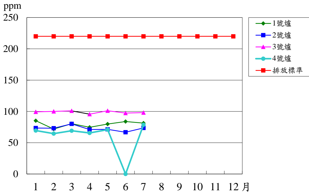
圖參之一(二)-2-113 年氮氧化物(NO x )排放監測值
