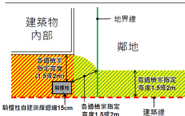
平面圖
