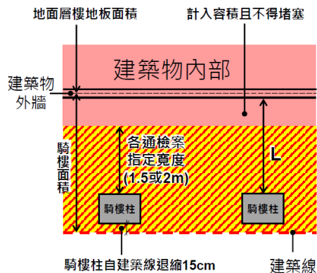
平面圖
