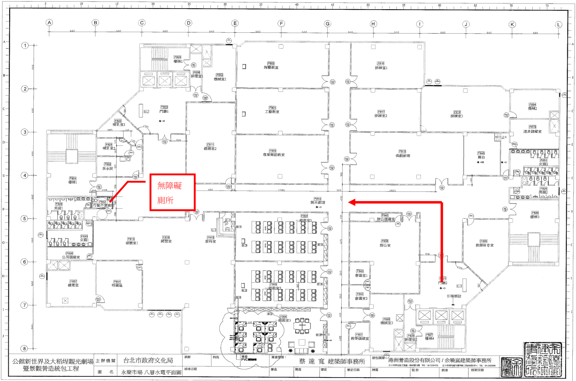
大稻埕戲苑 8 樓無障礙廁所空間、動線平面圖
